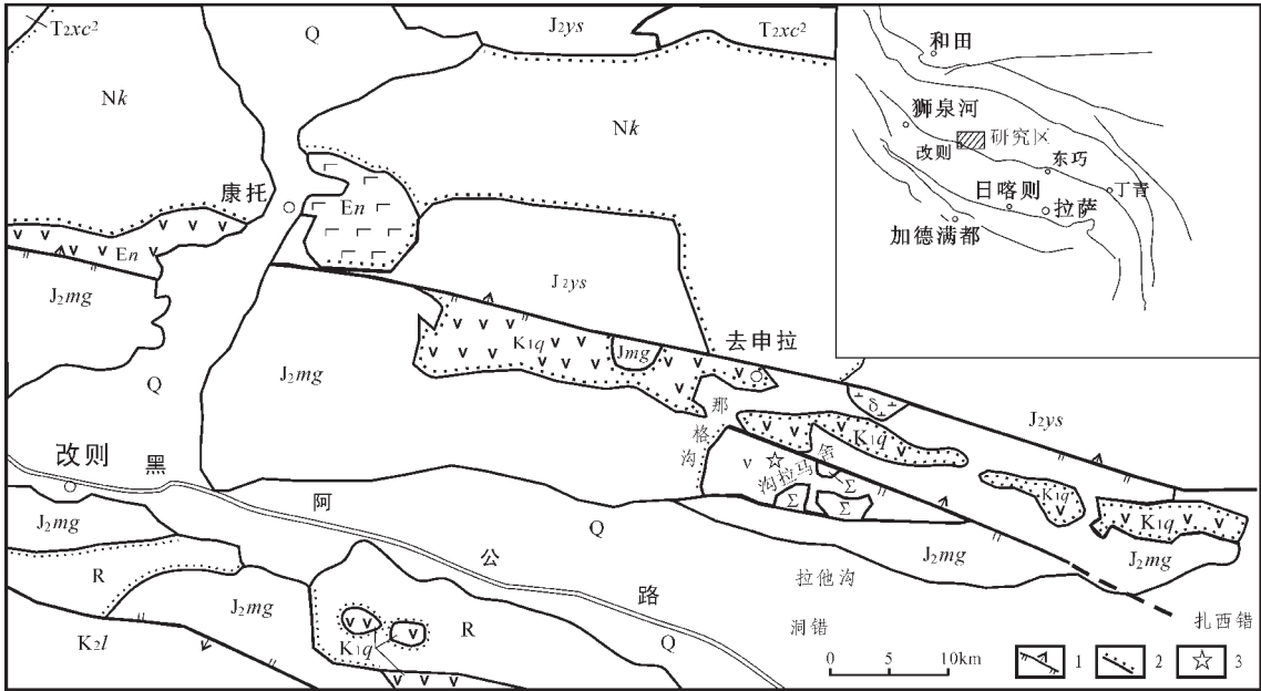
图1 班公湖—怒江蛇绿岩带西段舍马拉沟地质简图 Q—第四系;Nk—新近系;En—古近系;R—新近系古近系;K 2 l—上白垩统;K 1 q—下白垩统去申拉组; J 2 ys—中侏罗统;J 2 mg—中侏罗统木嘎岗日群;T 2 xc 2 —上三叠统;δ—燕山早期闪长岩;β—辉绿玢岩; ν—辉长岩;Σ—基性—超基性岩;1—断层;2—不整合界线;3—同位素测年样采样点
