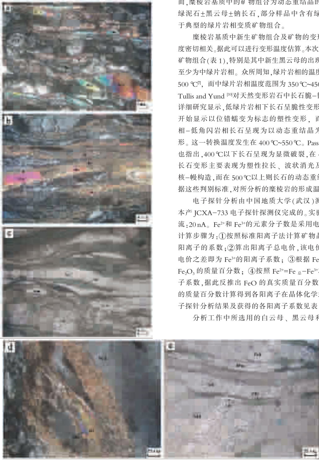
图 2 郯庐断裂带糜棱岩显微照片
