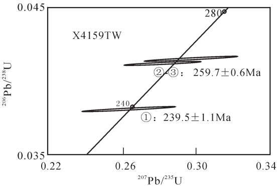
图 6 乌兰陶勒盖正长花岗岩锆石 U-Pb 一致曲线图 Fig.6 Zircon U-Pb concordia plot of the Ulan Tolgoi syenogranite
