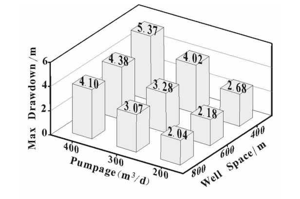
图 2 不同开采方案下开采井最大计算水位降深变化 Fig.2 Variation diagram of calculated maximum drawdowns in different scenarios
