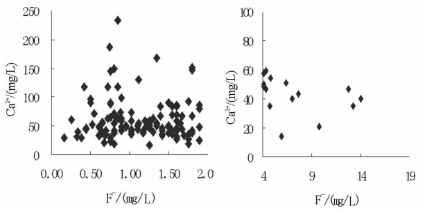
图 4 氟离子含量与钙离子含量的散点关系图 Fig.4 Scatter diagram of F^- and Ca^{2+} content
