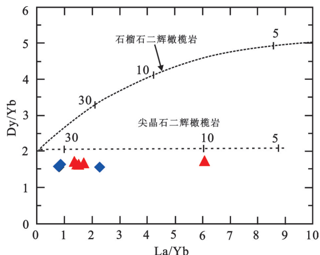
图 14 玄武岩 Dy/Yb—La/Yb 图解 (据文献[52]修改)
