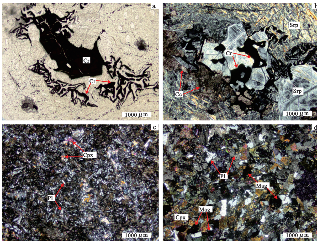
图4 木哈塔依蛇绿混杂岩样品号镜下照片
