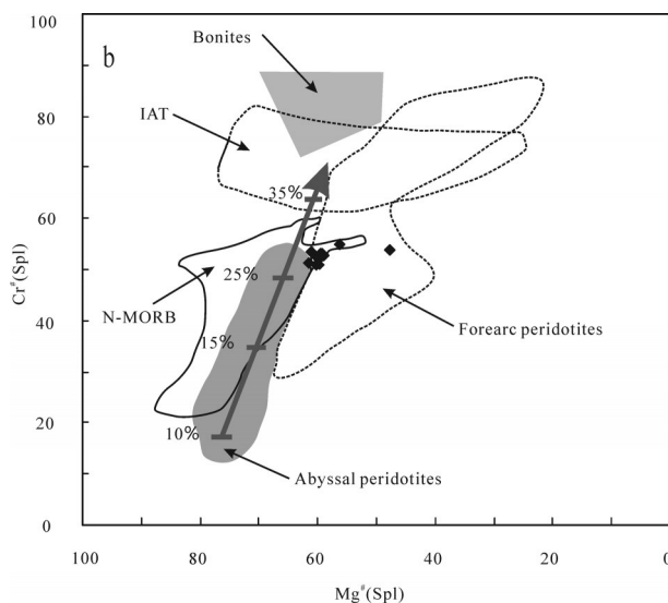
图5 方辉橄榄岩尖晶石Mg # -Cr # 判别图 (深海地幔橄榄岩、正常洋脊玄武岩和玻安岩来自文献[28];弧前地幔橄榄岩来自文献[29];带十字叉的箭头代表主体地幔橄榄岩部分熔融百分比来自文献[30])
