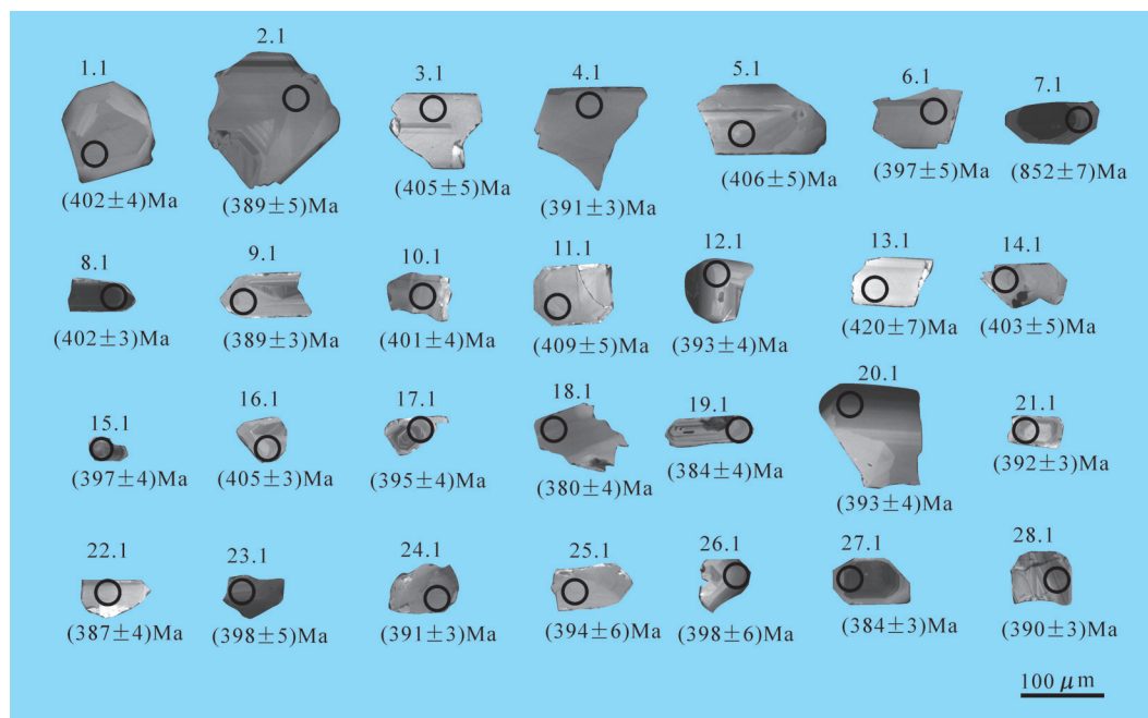
图9 木哈塔依蛇绿混杂岩中玄武岩的锆石阴极发光图像
