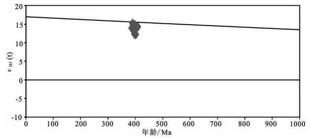
图11 玄武岩锆石的 \epsilon_{\text{Hf}}(t) 与锆石 U-Pb 年龄关系图 Fig.11 Plot of \epsilon_{\text{Hf}}(t) versus U-Pb age of zircon of basalt
