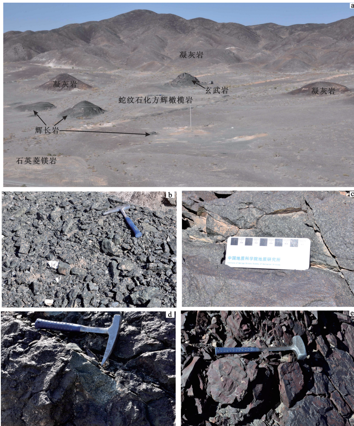
图3 木哈塔依蛇绿混杂岩野外产状
