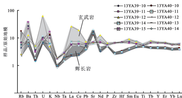
图8 辉长岩和玄武岩的微量元素原始地幔蛛网图(底图据文献[31]修改)
