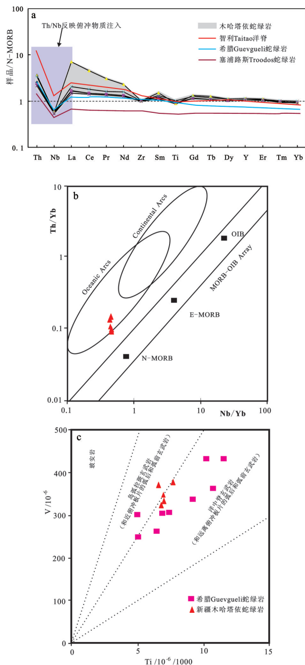
图 13 木哈塔依蛇绿混杂岩大地构造判别图
