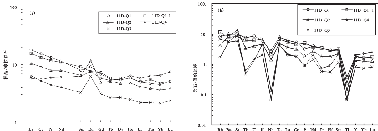
图3 红柳沟稀土元素球粒陨石标准化分布型式图(a)和微量元素原始地幔标准化蛛网图(b)
