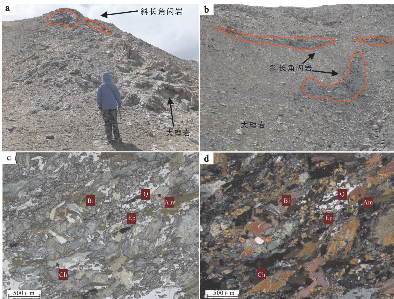
图2 斜长角闪岩野外及镜下特征
