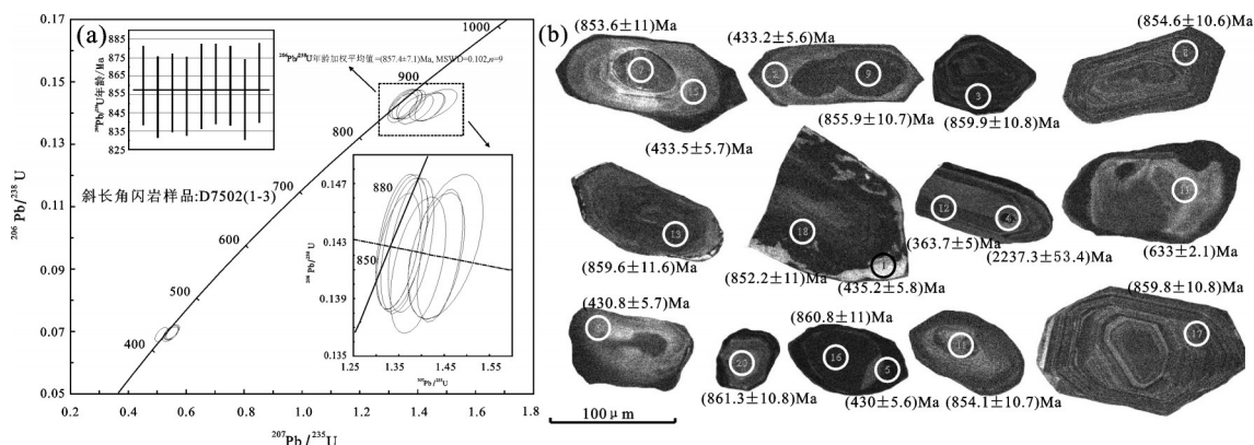
图3 斜长角闪岩U-Pb年龄谐和图(a)和部分锆石阴极发光图(b)
