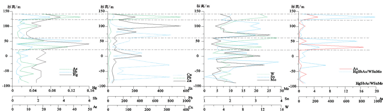
图4 姜里金矿区ZK11-2 钻孔元素轴向变化规律图
