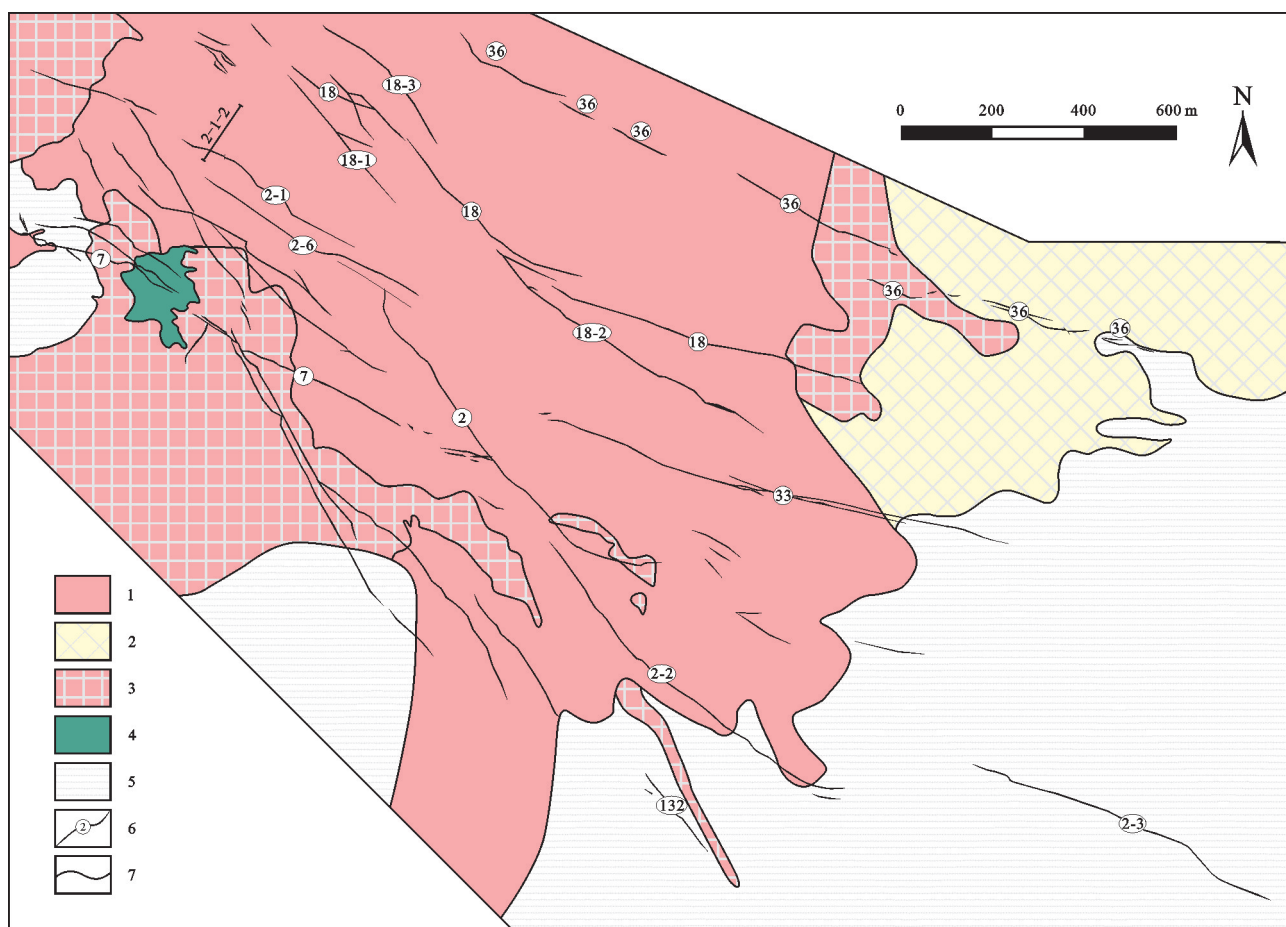
图2图古日格金矿区地质图(据[16]修改)
