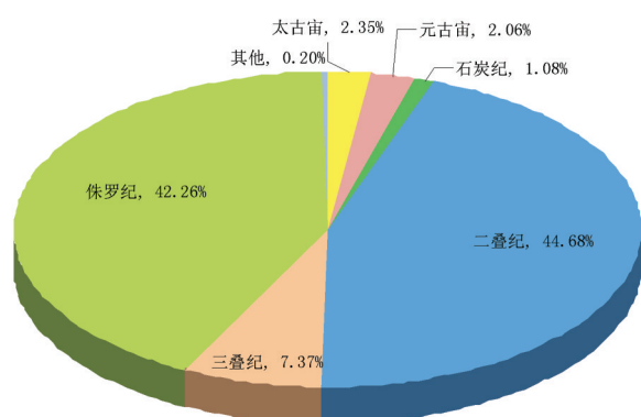
图4 中国不同成矿时代接触变质型(隐晶质石墨矿)资源储量分布比例
