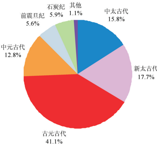
图3 中国不同成矿时代区域变质型晶质石墨矿资源储量分布 (资料来源于各省2016年资源储量通报) Fig.3 Proportion of resource reserves distribution of crystalline graphite deposits in different metallogenic epochs in China
