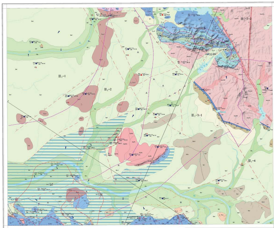
图2 莱芜市幅1:50 000水文地质图
