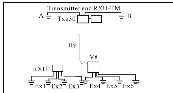
图3 CSAMT法V8(一主一辅)网络化野外作业方式示意图
