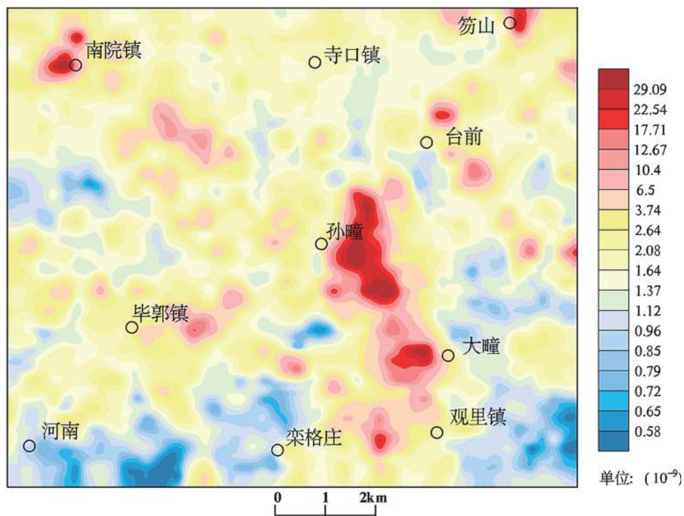
图2 毕郭幅金元素地球化学图
