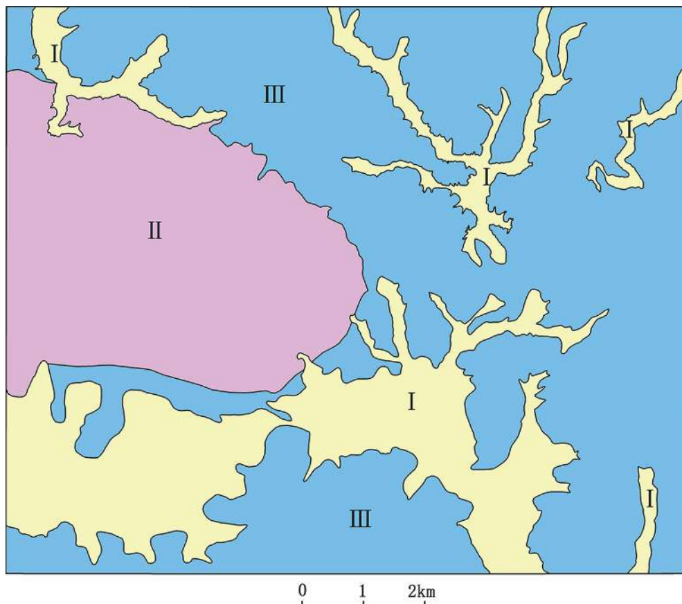
图3 毕郭幅地质分区图
