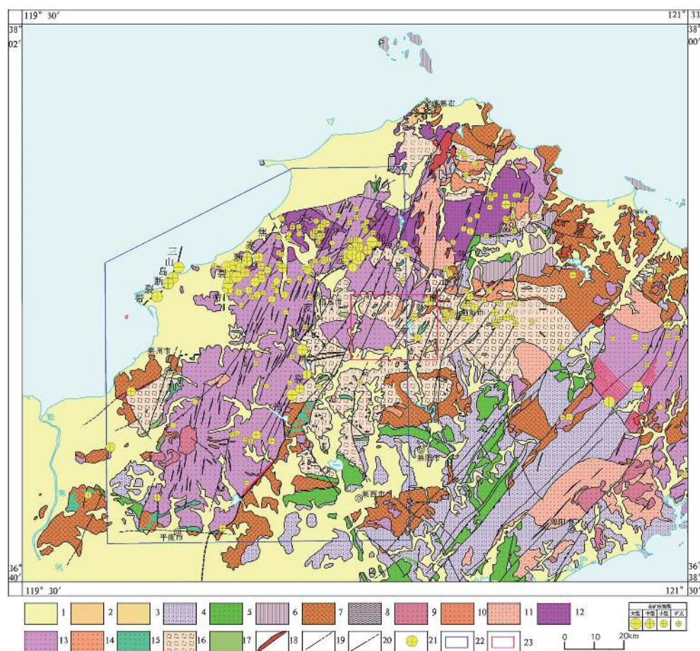
图 1 山东莱州-招远整装勘查区区域地质简图
