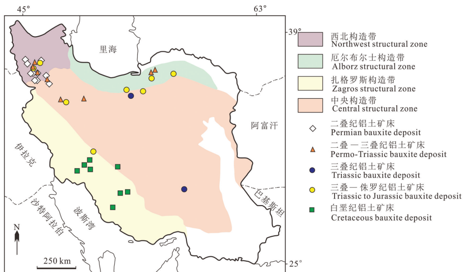
图8 伊朗铝土矿分布图(据 Abedini et al., 2020)
