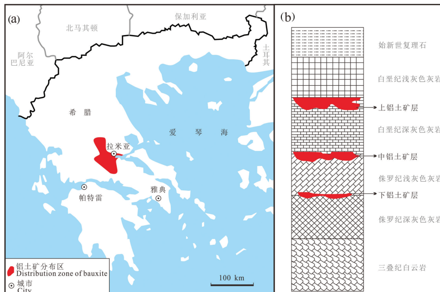
图6 希腊铝土矿分布区及典型含铝土矿层剖面(据Abedini et al., 2020)
