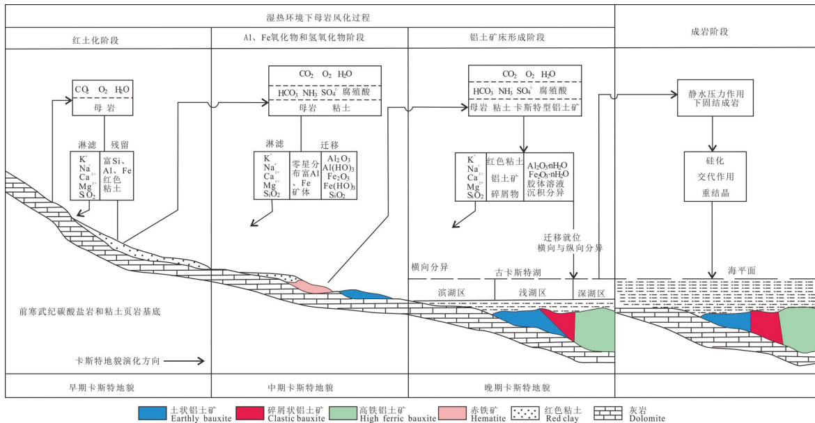
图5 岩溶型铝土矿成矿模式 (据 Li et al., 2020)
