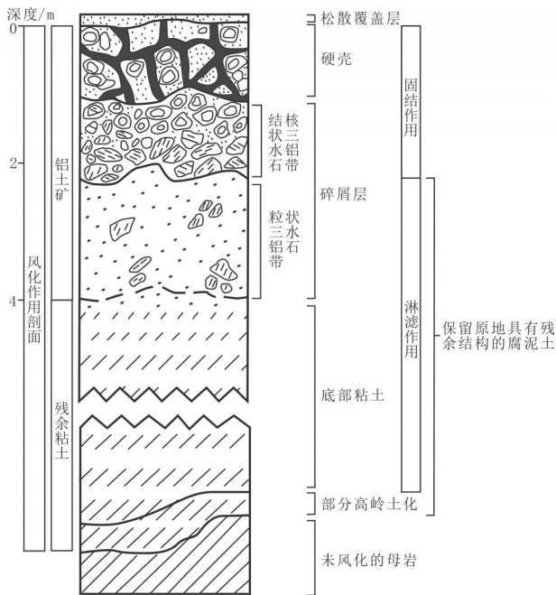
图2 典型红土型铝土矿剖面
