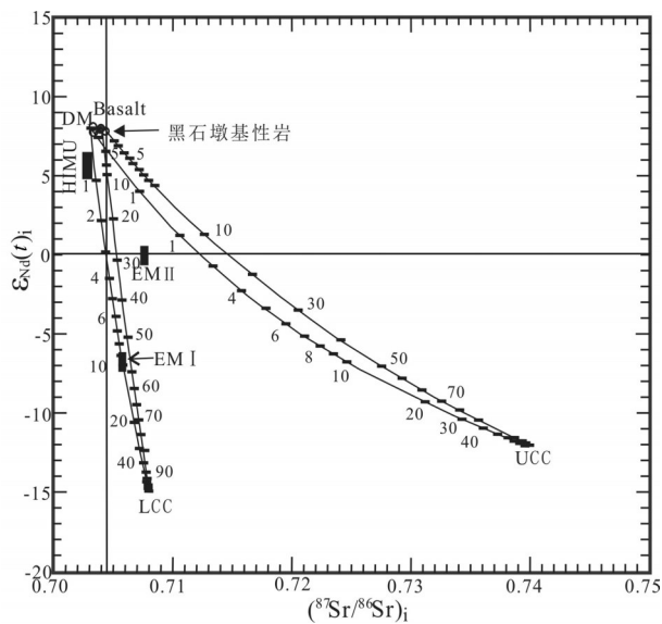
图9 黑石墩基性岩( ^{87}\text{Sr}/^{86}\text{Sr} ) -\varepsilon_{\text{Nd}}(t) 图解
