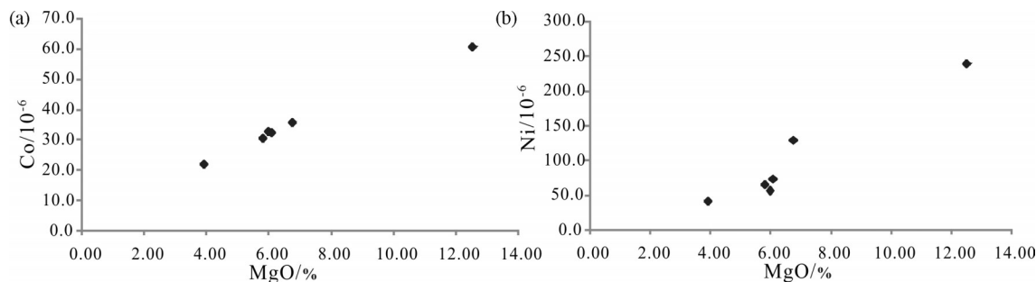
图7 黑石墩基性岩 MgO-Co 图解(a)和 MgO-Ni 图解(b)
