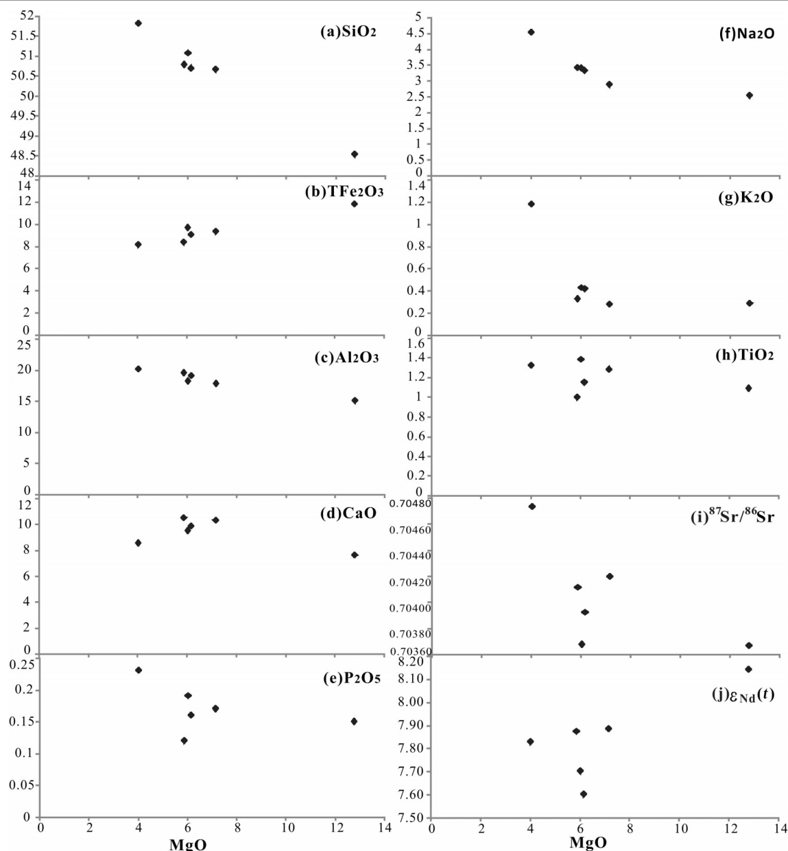
图4 黑石墩基性岩哈克图解(除 \varepsilon_{\text{Nd}}(t) 值外,其他单位均为%)
