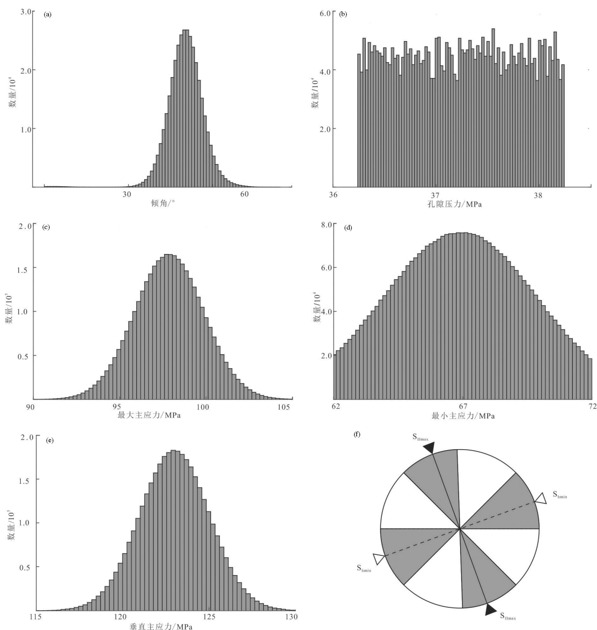
图2 蒙特卡洛模拟参数分布图
