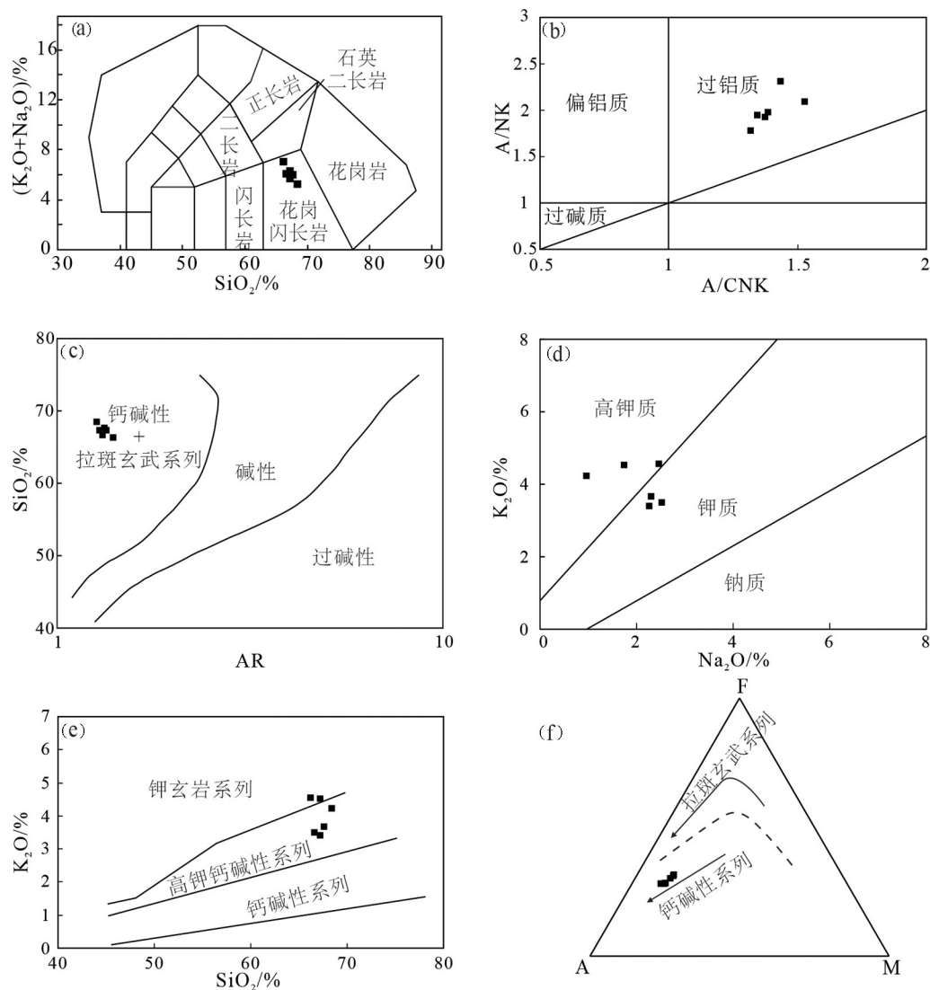
图6 黑云母花岗闪长岩主量元素判别图
