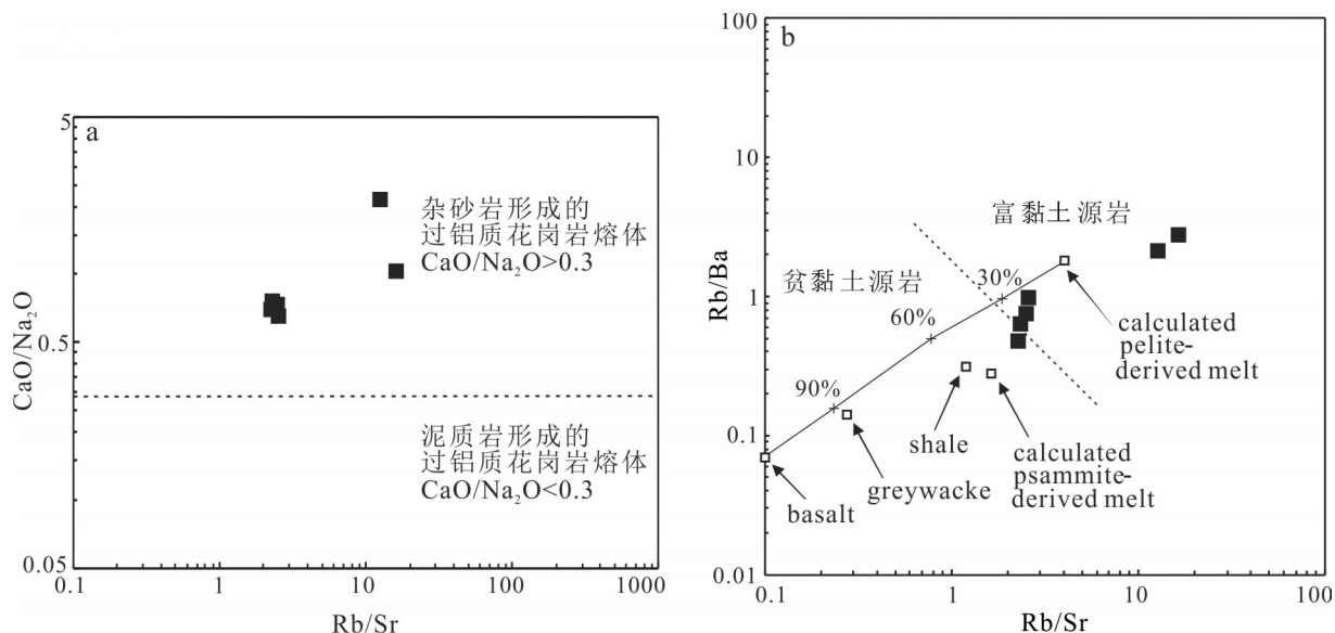
图 10 大湖塘黑云母花岗闪长岩的源岩判别图解(据 Sylvester, 1998)
