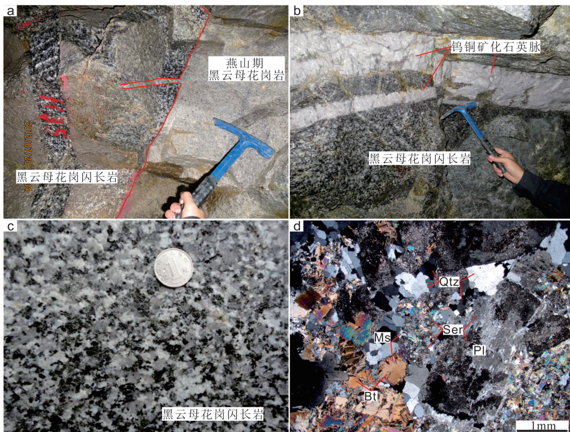
图3 大湖塘黑云母花岗闪长岩产出特征及岩石标本照片
