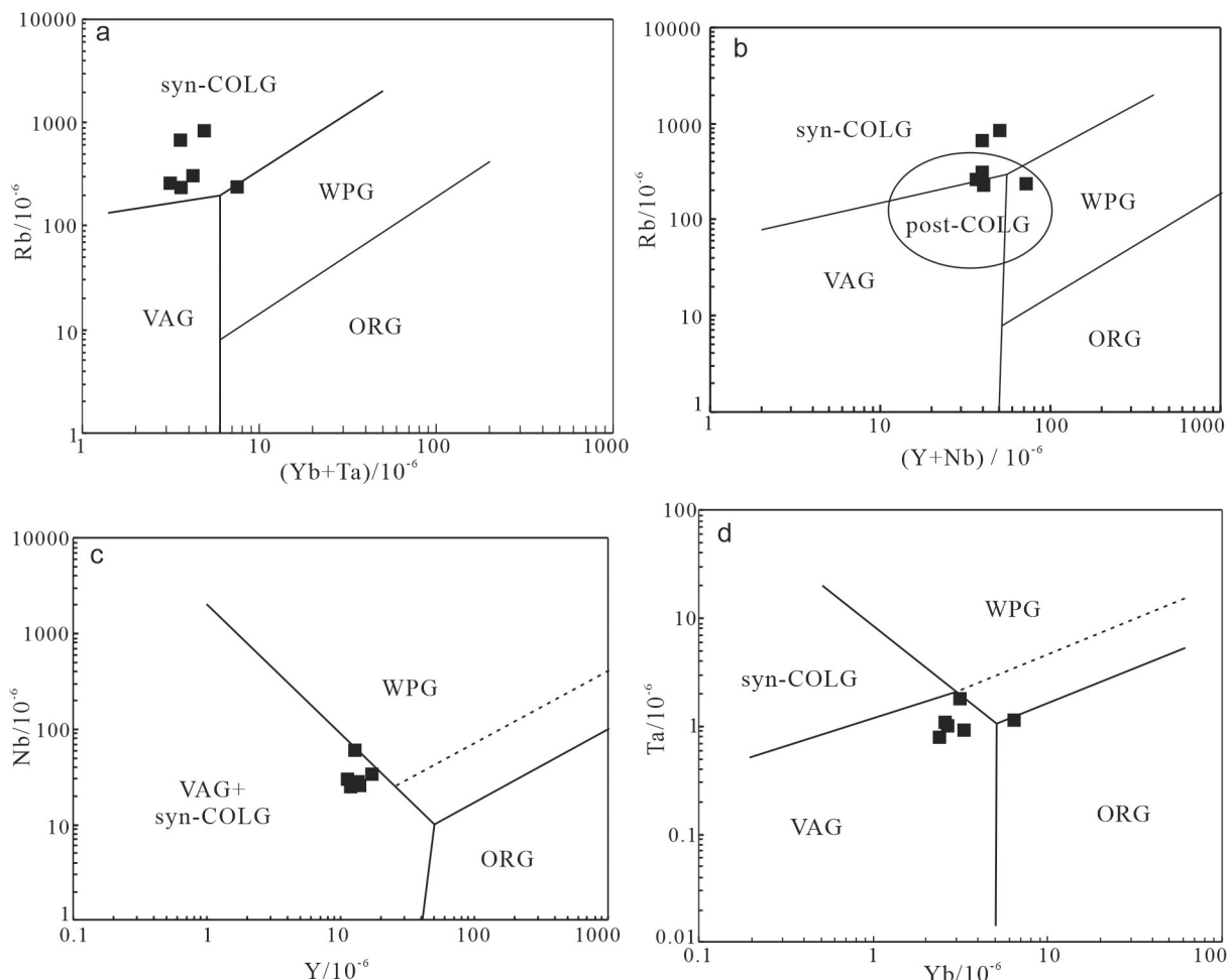
图 11 大湖塘黑云母花岗闪长岩构造环境判别图(底图据 Pearce et al., 1984)
