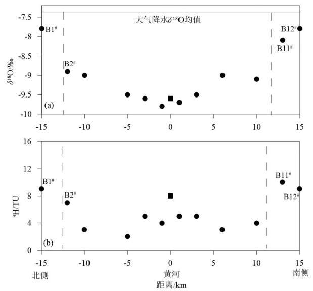
图5 济阳剖面B-B'地下水的同位素变化
