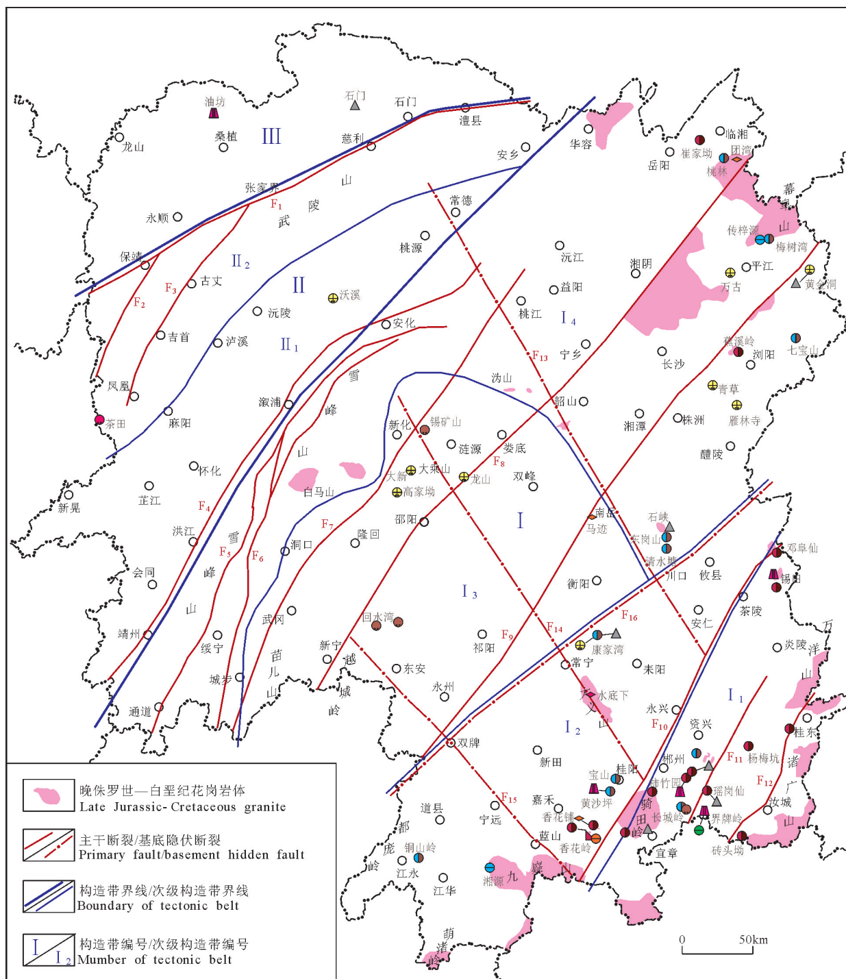
图4 晚侏罗世—早白垩世早期内生热液成矿期构造格局(据柏道远等,2020;断裂名称及矿床类型同图1) I—湘中—湘东构造岩浆带: I 1 —炎陵—汝城冲断褶皱隆带, I 2 —宁远—桂阳拗陷带, I 3 —邵阳拗陷带, I 4 —雪峰东南部构造岩浆隆起带; II—雪峰西部构造带: II 1 —怀化—桃源冲断带, II 2 —武陵断弯褶皱带; III—湘西北褶皱带
