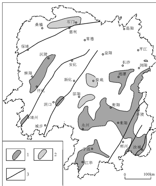
图11 晚三叠世—早侏罗世构造古地理格局与成矿
