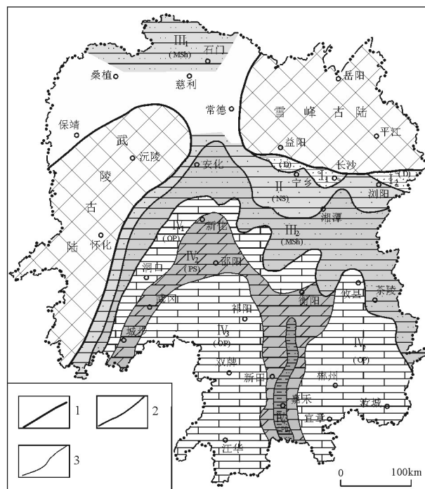
图10 晚泥盆世锡矿山区构造古地理格局
