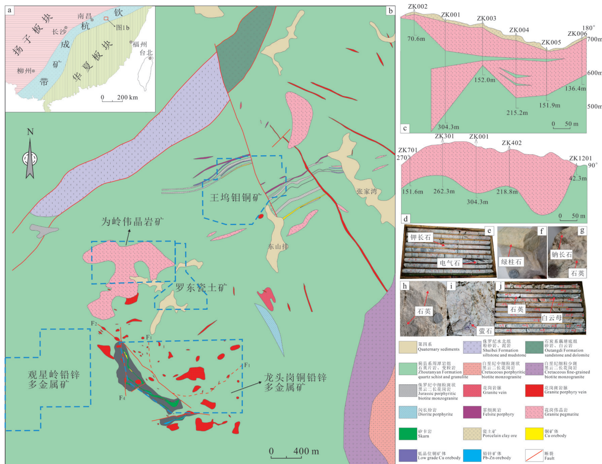
图1 钦杭成矿带构造示意图(a)、龙头岗—为岭矿区地质图(b)、0号勘探线剖面图(c)、纵剖面图(d)、为岭及周边伟晶岩野外照片(e-j)
