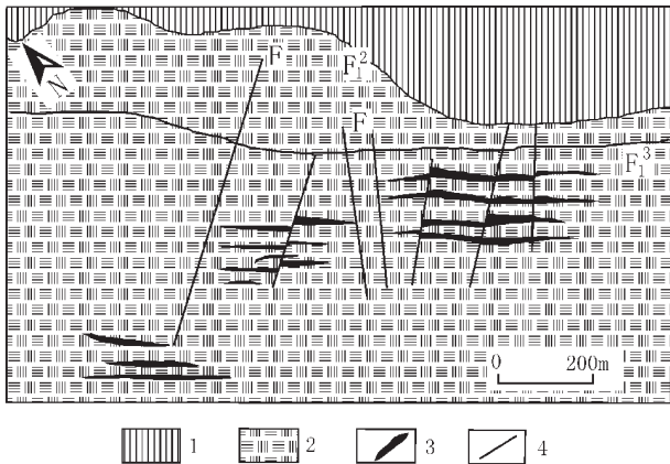
图1 陕西凤县八卦庙超大型金矿床矿区地质图 (据方维萱, 2000, 修编)
