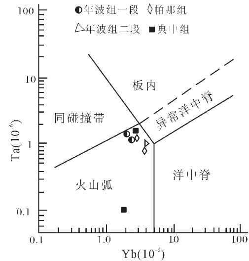
图 7 林子宗群火山岩 Yb—Ta 图解 Fig.7 Yb—Ta diagram for volcanic rocks of the Linzizong Group
