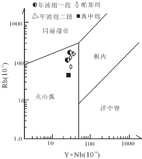
图 8 Rb—(Y+Nb)图解 Fig. 8 Rb—(Y+Nb) diagram
