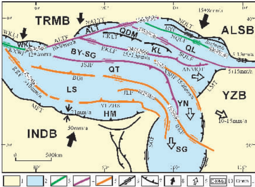
图 2 青藏高原大型走滑构造图
