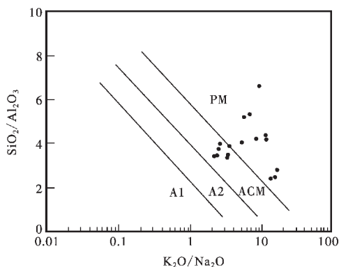
图3 K_2O/Na_2O-SiO_2/Al_2O_3 构造背景判别图解 (据参考文献[15])
