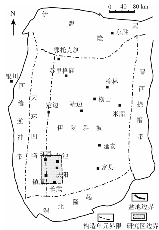
图 1 研究区构造位置略图 Fig.1 Structural location of the study area
