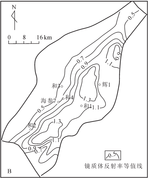
图 3 呼和湖凹陷镜质体反射率( R_o )平面分布图
