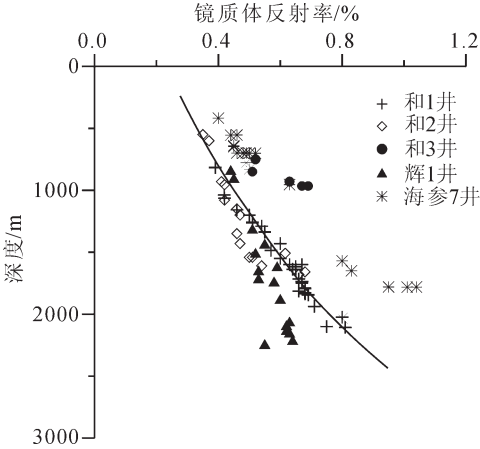
图 2 呼和湖凹陷镜质体反射率( R_o )与深度关系
