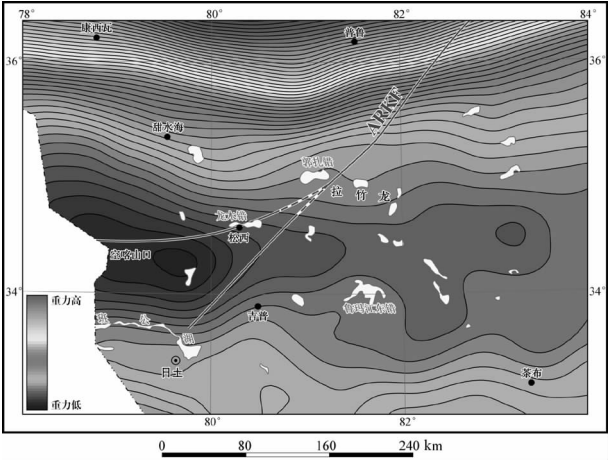
图 4 甜水海—郭扎错—日土一带的向上延拓 20 km 布格重力异常图
