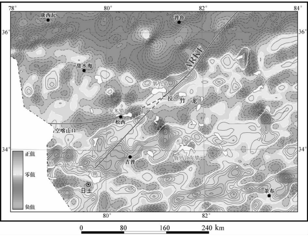
图 3 甜水海—郭扎错—日土一带重力异常 135^\circ 方向的水平导数图
