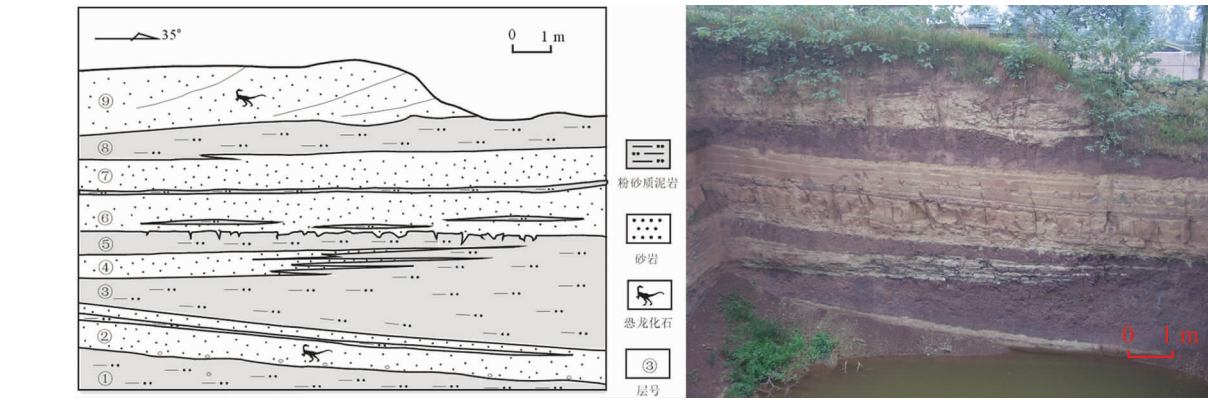
图 3 自贡恐龙博物馆内恐龙采坑中的地层剖面图和照片 Fig.3 Stratigraphic section and photo of dinosaur-collecting pit in the Zigong Dinosaur Museum
