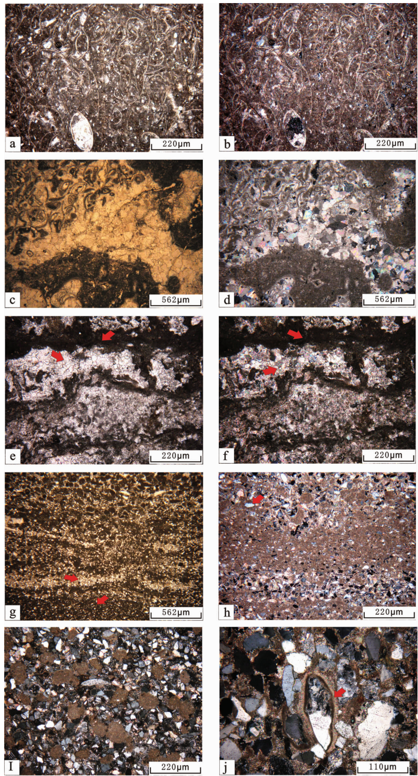
图版 II 介壳灰岩,藻叠层石灰岩显微特征(a,c,e 单偏光;b,d,f 正交偏光); 泥晶灰岩,砂质灰岩显微特征(g,i 单偏光;h,j 正交偏光)
