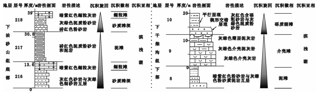
图 3 鲕粒滩和介壳滩沉积序列
