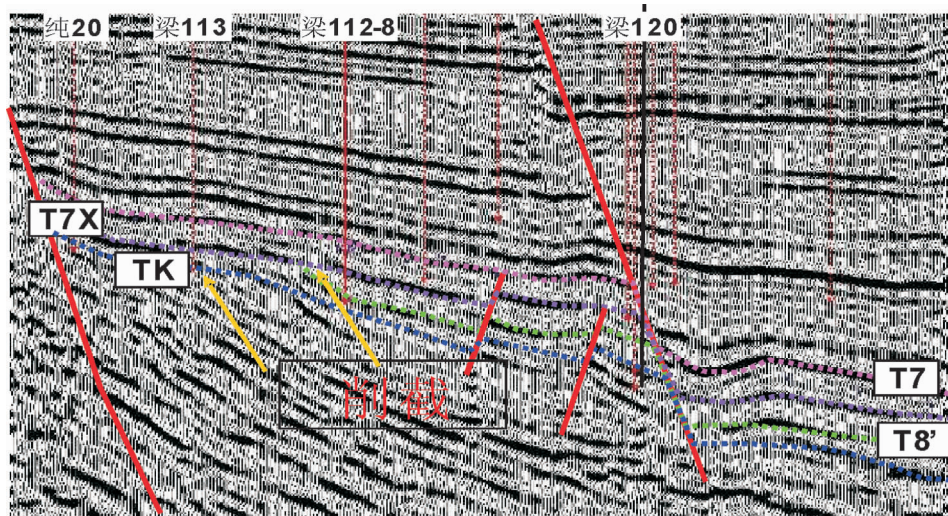
图 2 东营南坡过纯 20—梁 113—梁 112-8—梁 120 地震剖面图
