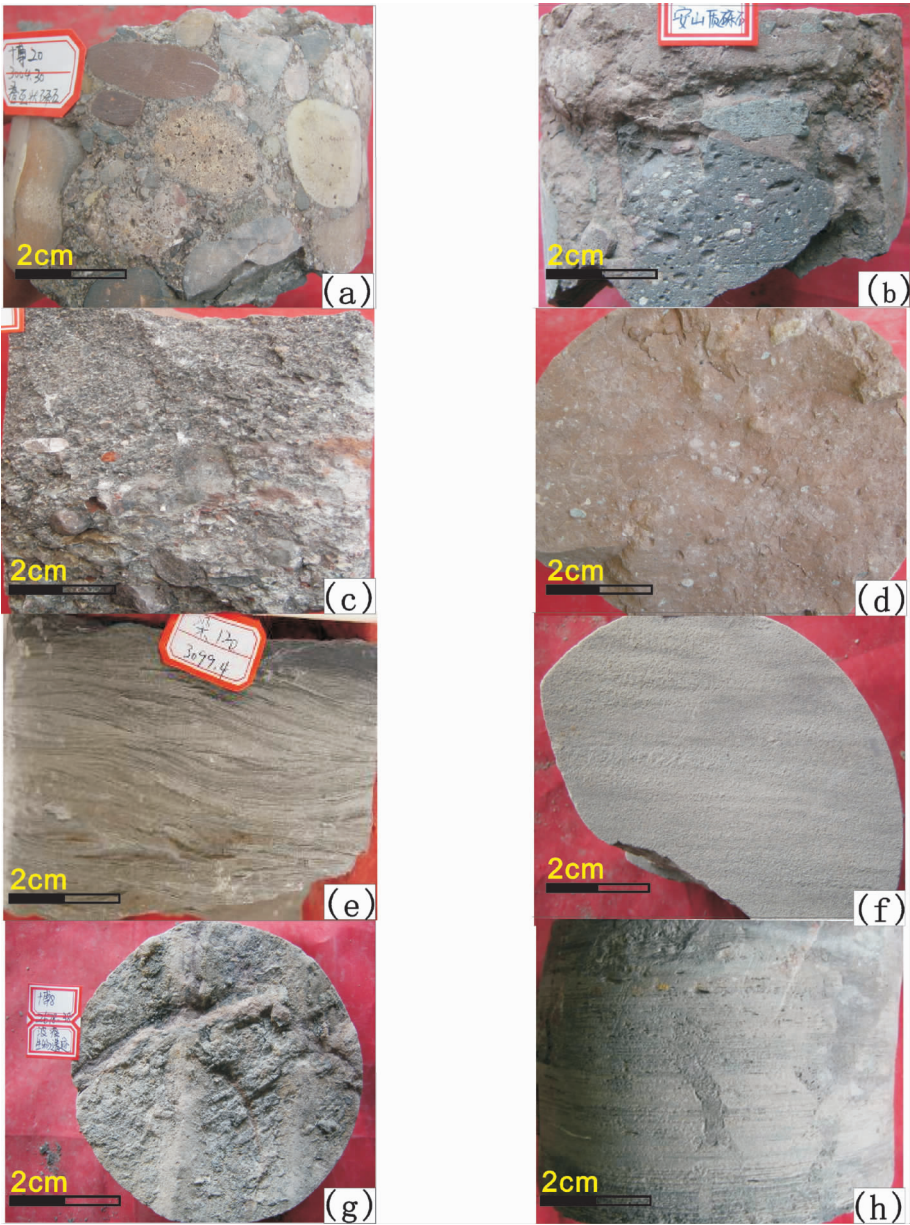
图 5 东营凹陷南坡沙四下亚段岩心照片
