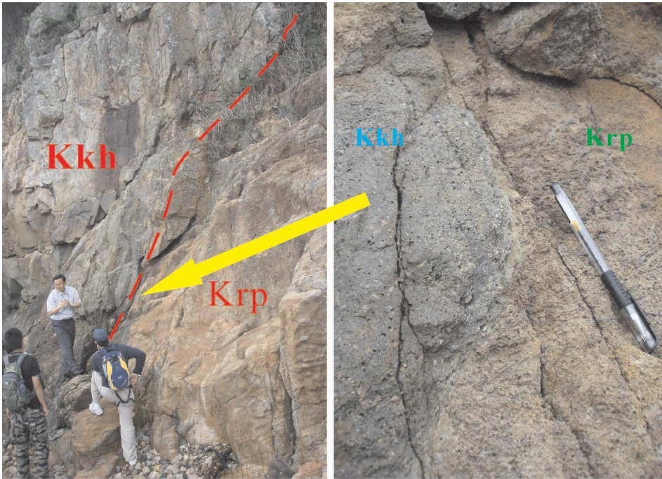
图 13 清水湾半岛龙虾湾粮船湾组(Kkh)与槟榔湾组(Krp)侵入接触关系(考察点:08HK107) 左图:粮船湾组与围岩槟榔湾组火山岩呈侵入接触关系,接触面陡;右图:粮船湾组出现较窄的灰绿色冷凝边,槟榔湾组棕红色流纹条带被接触面截断
