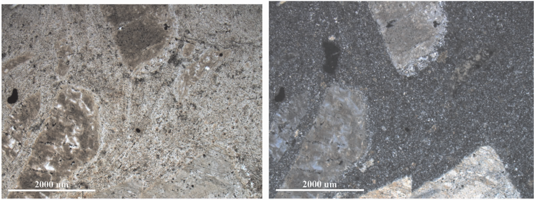
图 6 万宜水库西坝粮船湾组碎斑熔岩显微照片(样品:08HK204) 左图:碎斑熔岩含大量流纹条带,表面泥化的钾长石斑晶破碎成为碎斑(单偏光);右图:钾长石斑晶普遍发育珠边结构,基质中的流纹条带脱玻形成极细微的长英质集合体(正交偏光)
