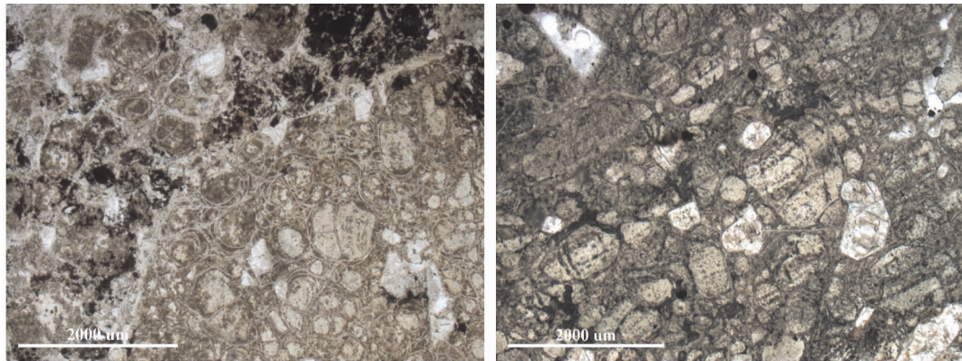
图 9 南果洲南部槟榔湾组(Krp)自碎角砾熔岩显微照片(样品:08HK126) 左图:角砾和胶结物均为流纹质熔岩,角砾具有清晰的珍珠构造(单偏光);右图:自碎角砾熔岩的胶结物由自形钾长石斑晶及具流动构造的基质组成(单偏光)
