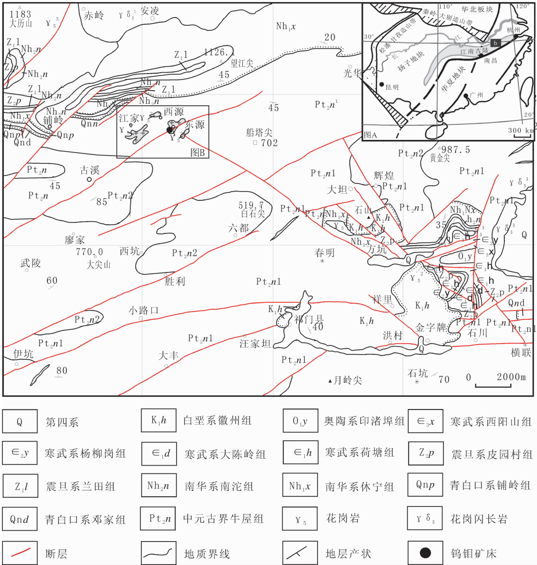
图 1 皖南祁门县东源钨钼矿区地质简图 [2]
