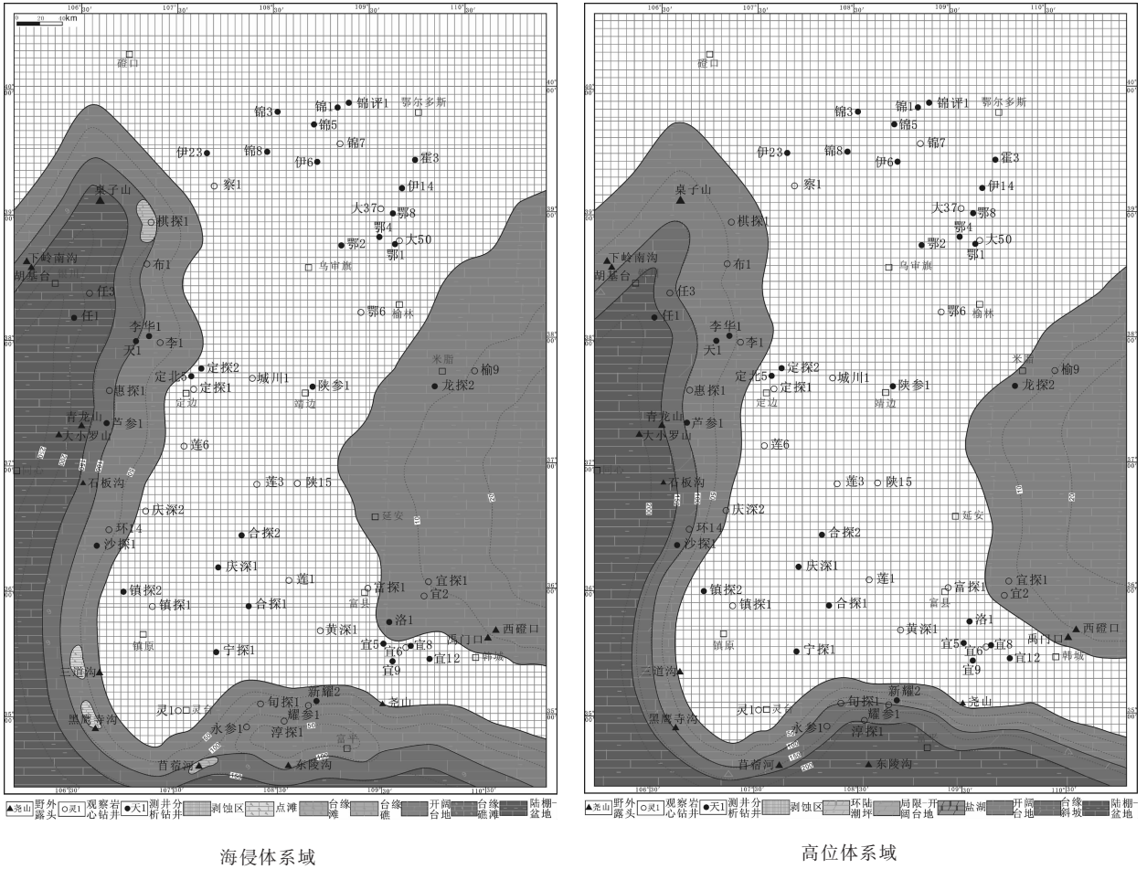
图 8 鄂尔多斯地区马家沟组 OSQ6 层序海侵体系域和高位体系域岩相古地理图
