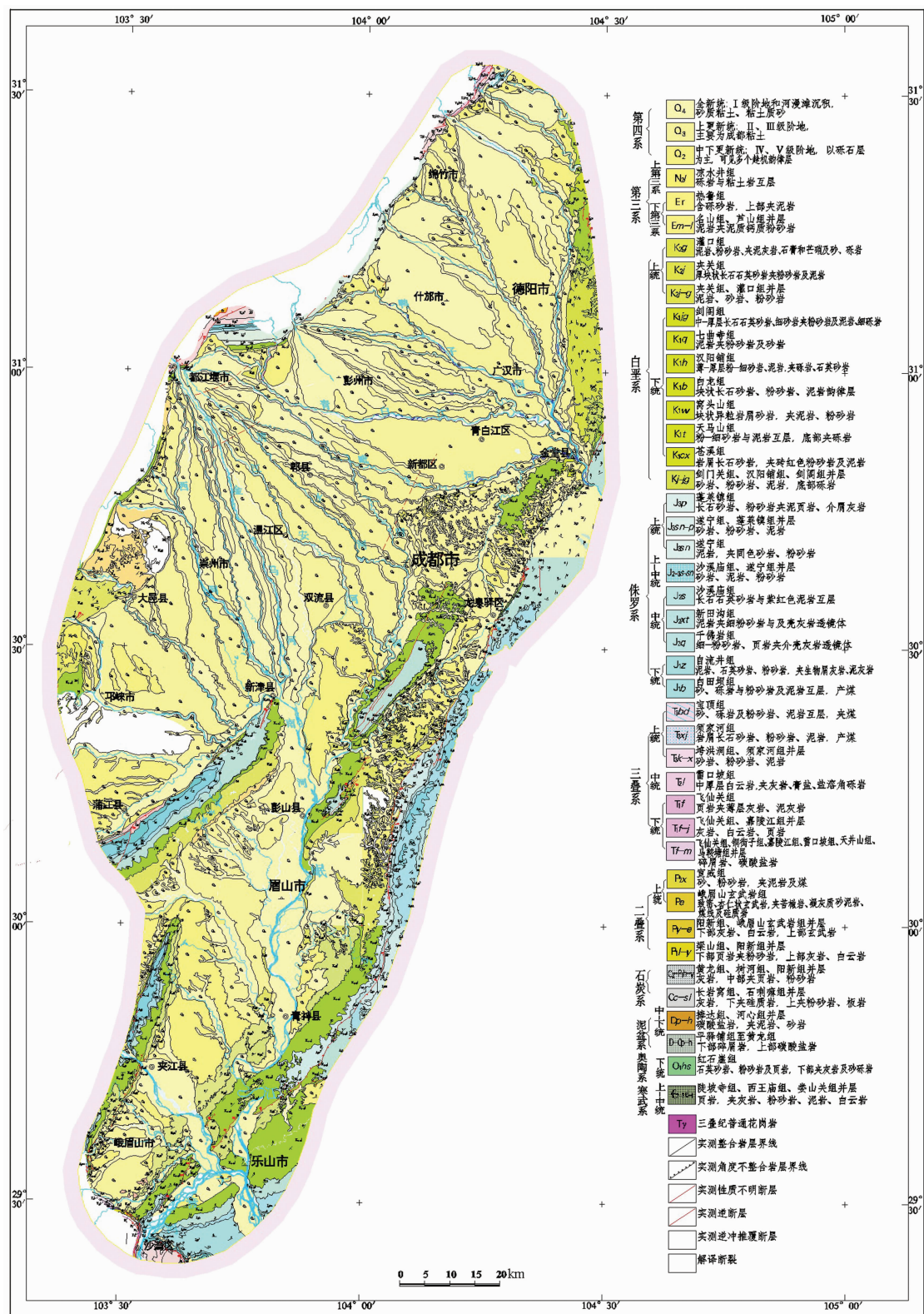
图 2 成都平原主要第四纪单元分布图 Fig.2 Distribution of main Quaternary units in Chengdu plain
