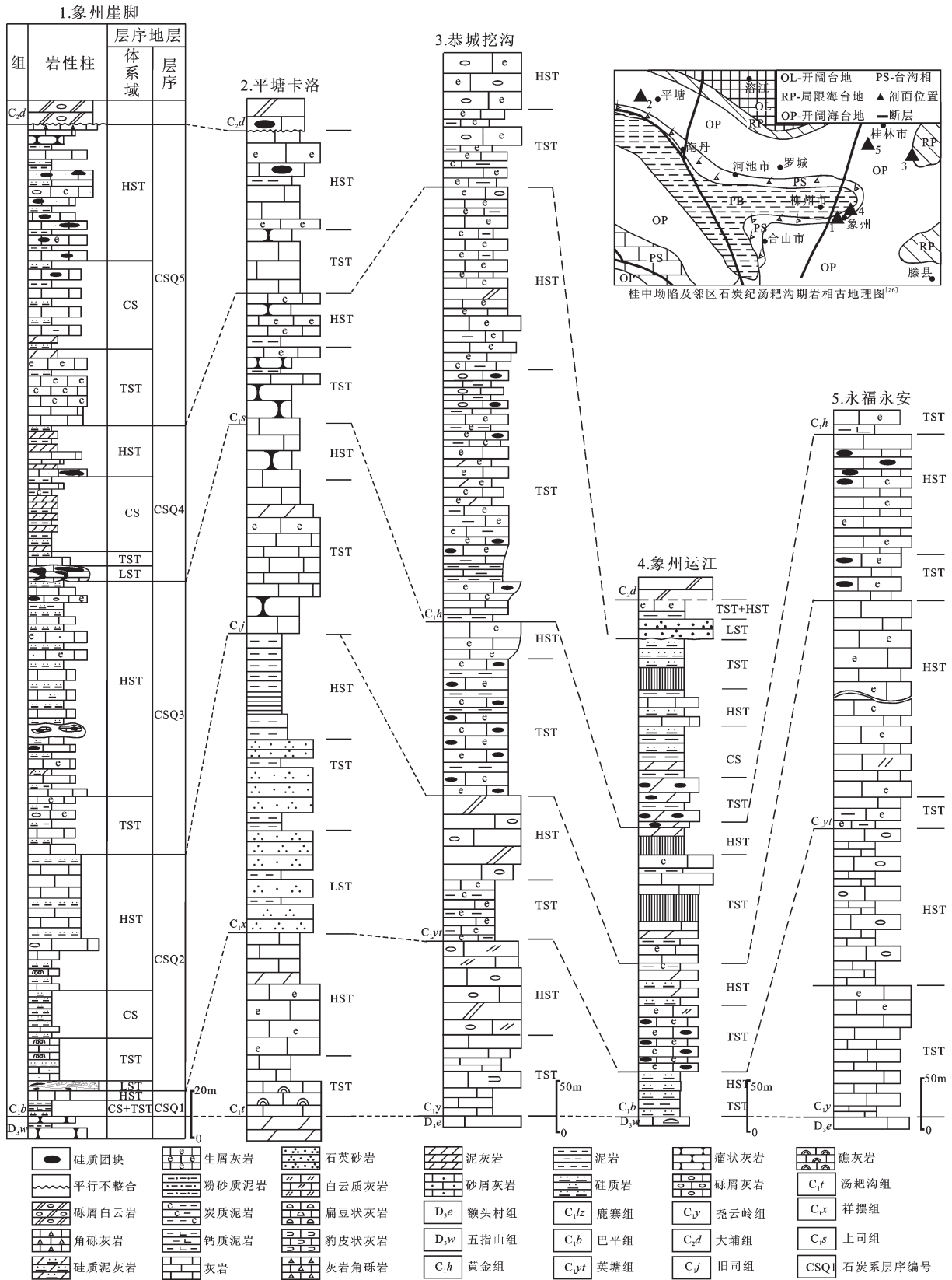
图5 不同相区早石炭世地层划分与对比
