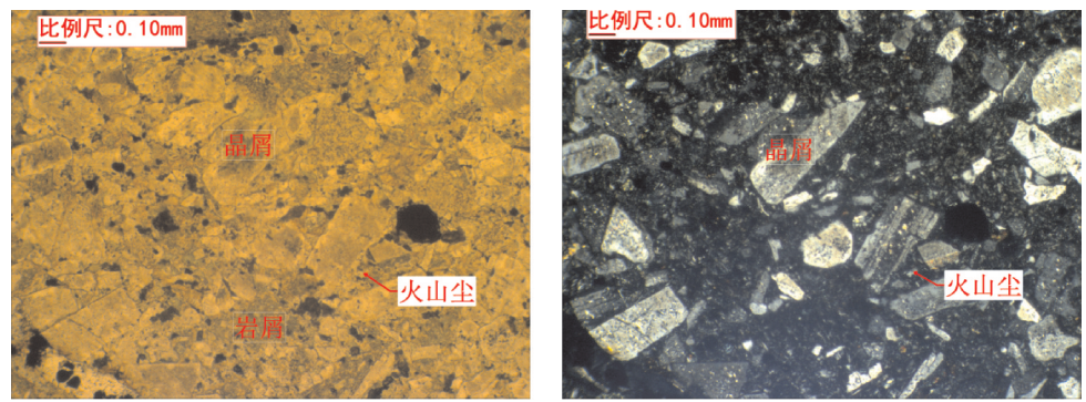
图3 幸福之路组凝灰岩镜下特征
