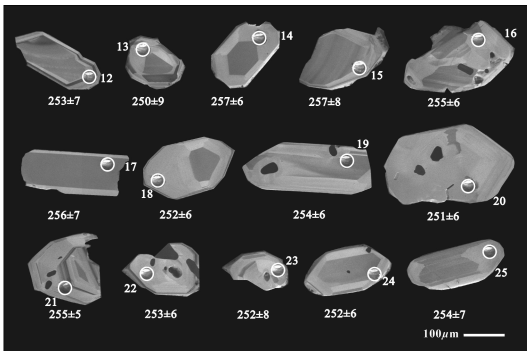
图4 幸福之路组凝灰岩的锆石阴极发光图像和 ^{206}\text{Pb}/^{238}\text{U} 年龄(Ma)
