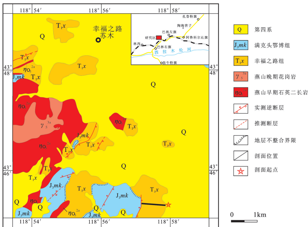
图1 幸福之路地区地质简图
