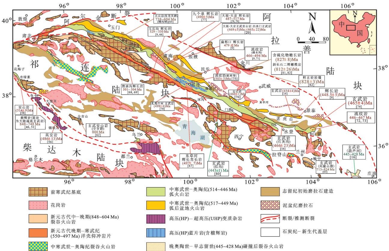
图2 祁连山地质略图(兼示主要火山岩带位置及其年龄)
