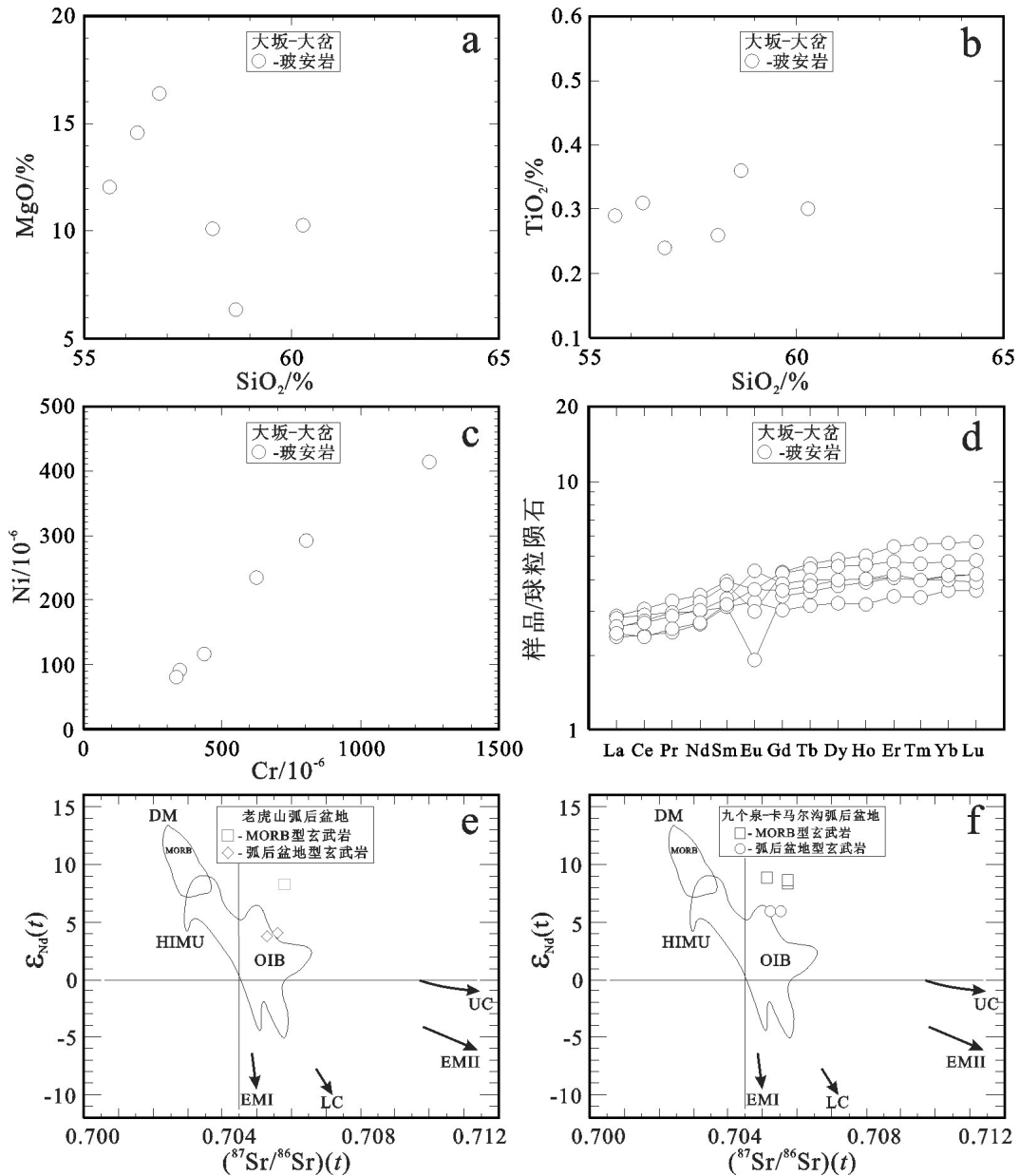
图22 北祁连山大坂—大岔地区玻安岩的a—MgO - SiO 2 图解, b—TiO 2 -SiO 2 图解, c—Ni—Cr图解和d—REE球粒陨石(据 [201])标准化蛛网图; e和f—老虎山和九个泉—卡马尔沟弧后盆地中玄武岩的ε Nd (t) - 87 Sr/ 86 Sr(t)图解, 图解据[185]
