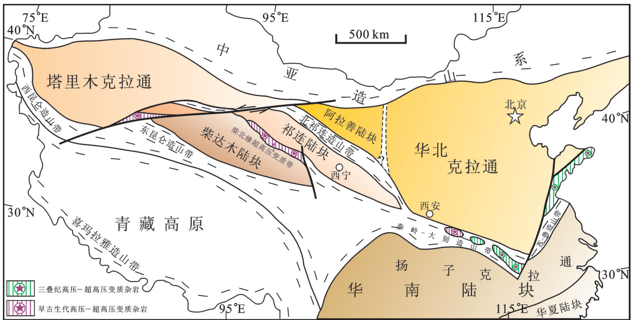
图1 中国大地构造格架简图(示主要前寒武纪克拉通、陆块和显生宙造山带)
