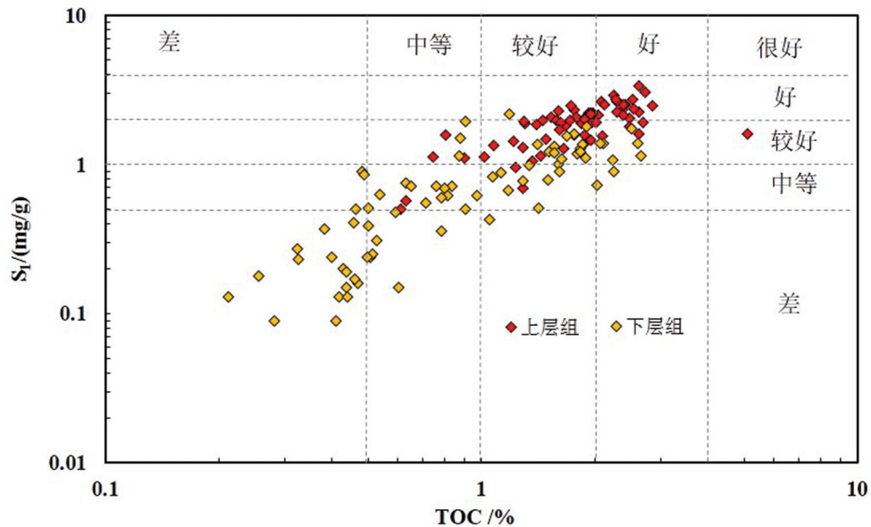
图9 青一段泥岩有机质丰度评价图
