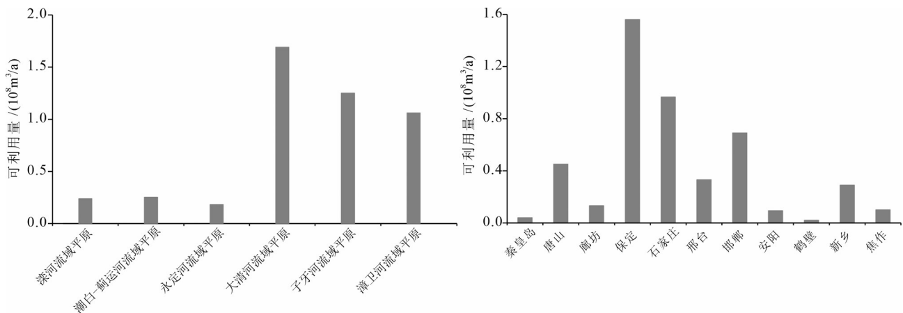
图9 深层水可利用量(a,按地下水资源区;b,按行政区)
