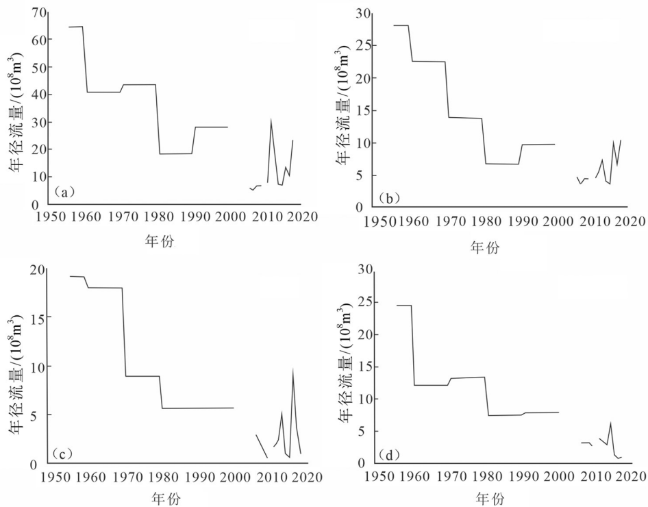
图4 海河流域主要河流出山口实测径流量
