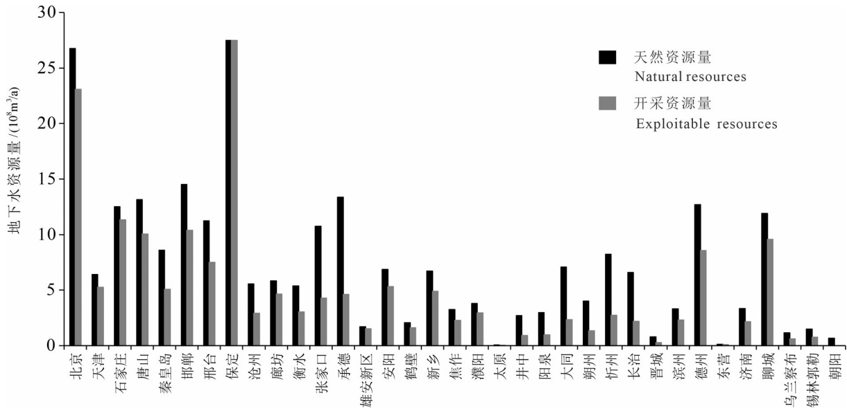
图8 海河流域地下水资源量(按行政区)
