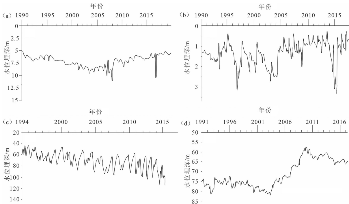
图6 海河流域平原地下水位动态曲线 a—潮白河冲洪积扇-浅层水-山前平原;b—沧州市-浅层水-中东部平原; c—中东部平原-衡水景县;d—沧州市-深层水-城市区
