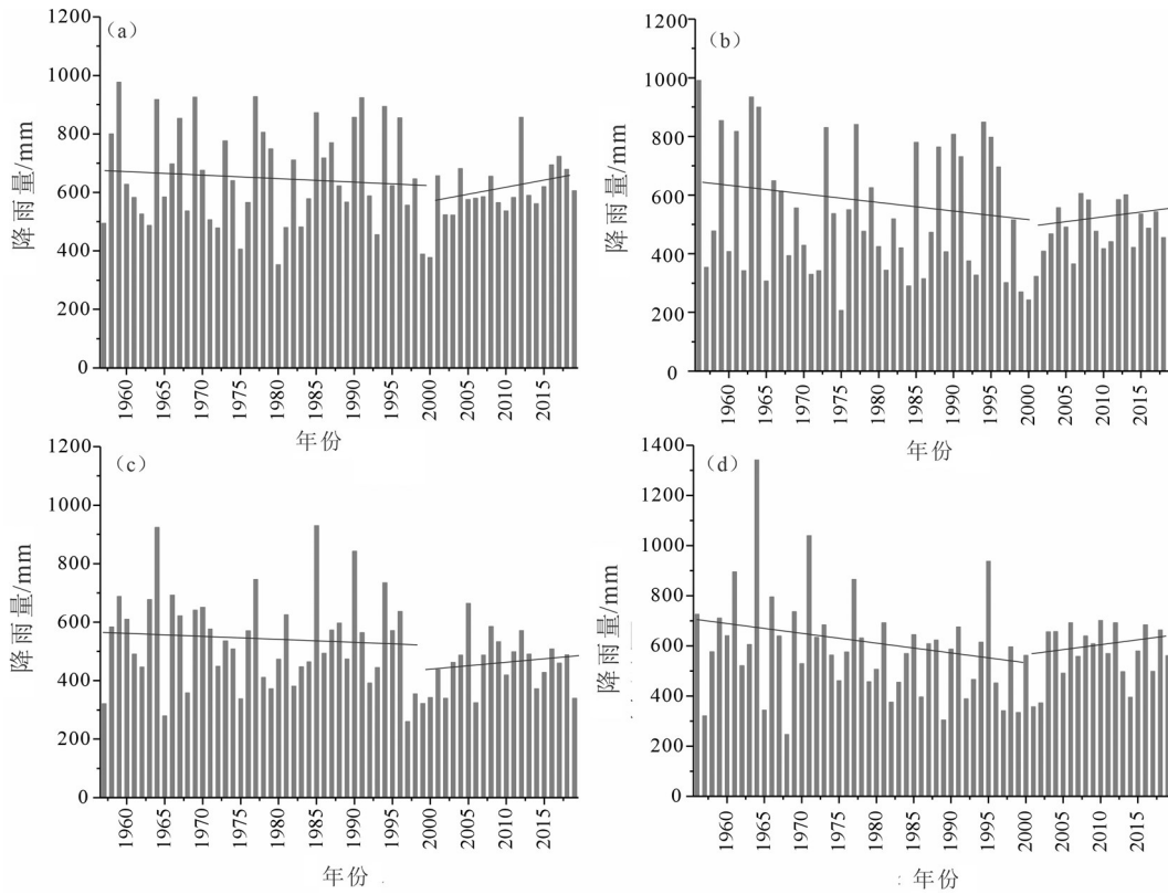
图3 海河流域降水量变化趋势 a—密云站-山区;b—保定站-山前平原;c—饶阳站-中部平原;d—黄骅站-滨海平原
