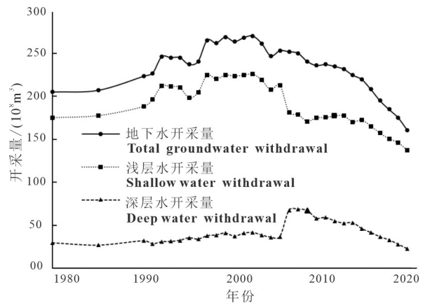
图5 海河流域地下水开采量变化趋势
