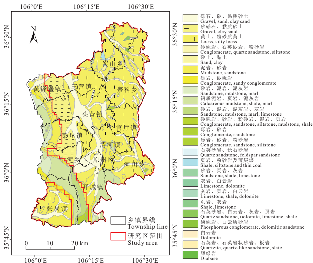
图 6 研究区地质简图
