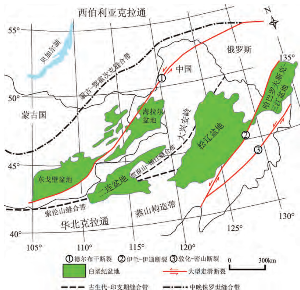
图9 东北亚中生代盆地与大型走滑断裂构造略图
