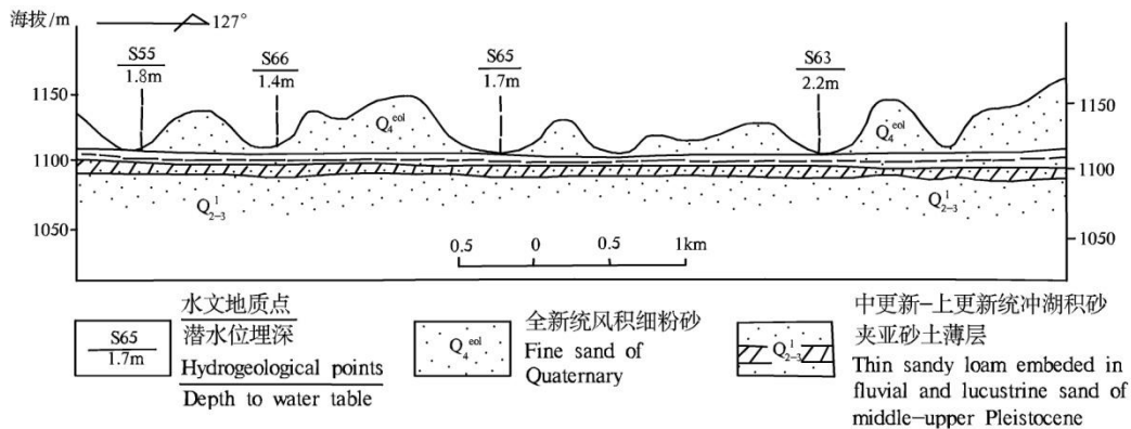
图 4 沙漠中典型水文地质剖面图
