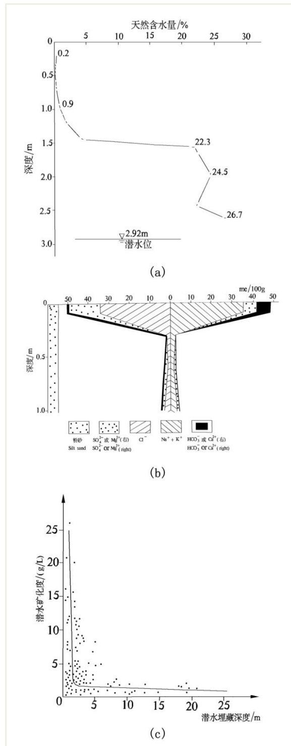
图 2 含水率剖面图 (a)、水化学剖面图 (b)、矿化度与地下水埋深关系图 (c)
