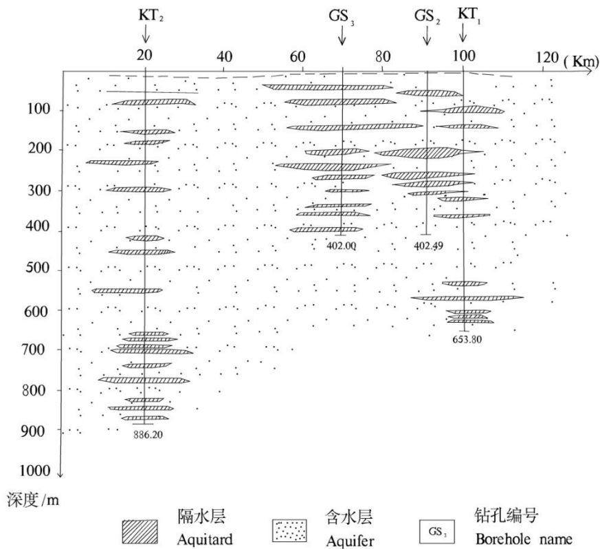
图 5 沙漠区含水层与隔水层空间展布图
