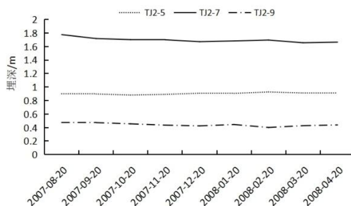
图 3 地下水浅埋区地下水动态图
