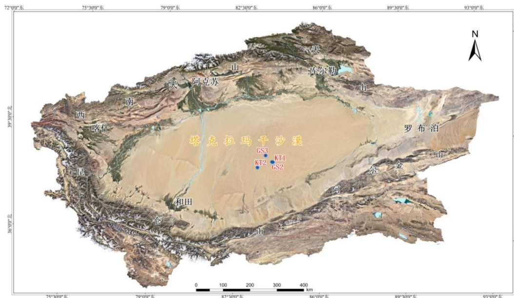
图 1 塔克拉玛干沙漠地理位置图以及沙漠中的水文地质深孔
