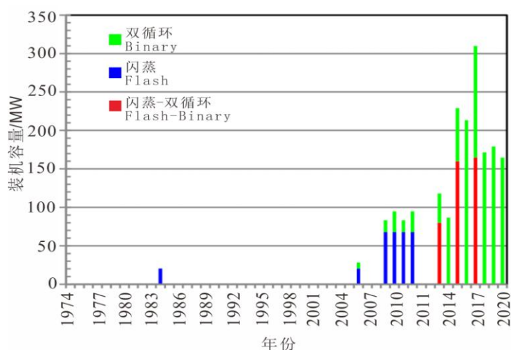
图5 按工厂类型每年增加的地热发电装机容量（据 Serpen et al.,2022）
