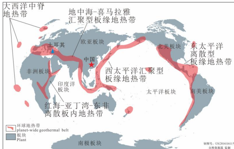
图1 全球高温地热带分布 (据何治亮等, 2017)
