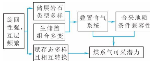
图 2 煤系气基本地质特点及其控制关系
