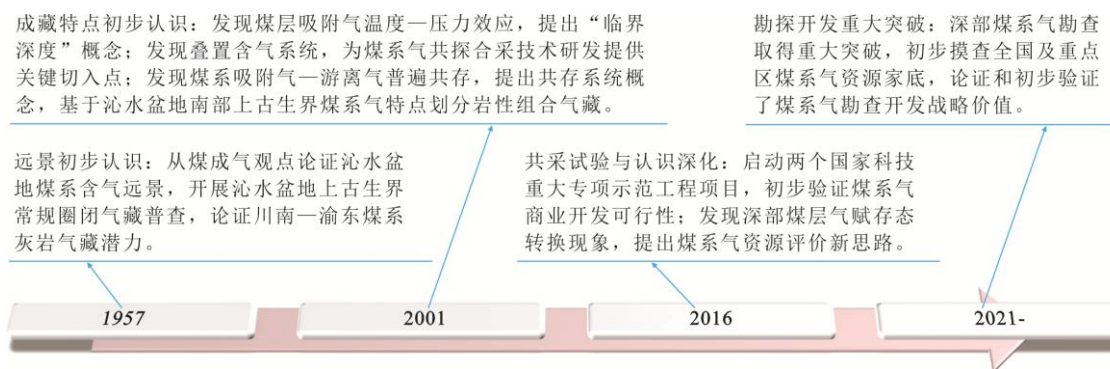
图 1 中国煤系气地质调查与勘探开发试验简史
