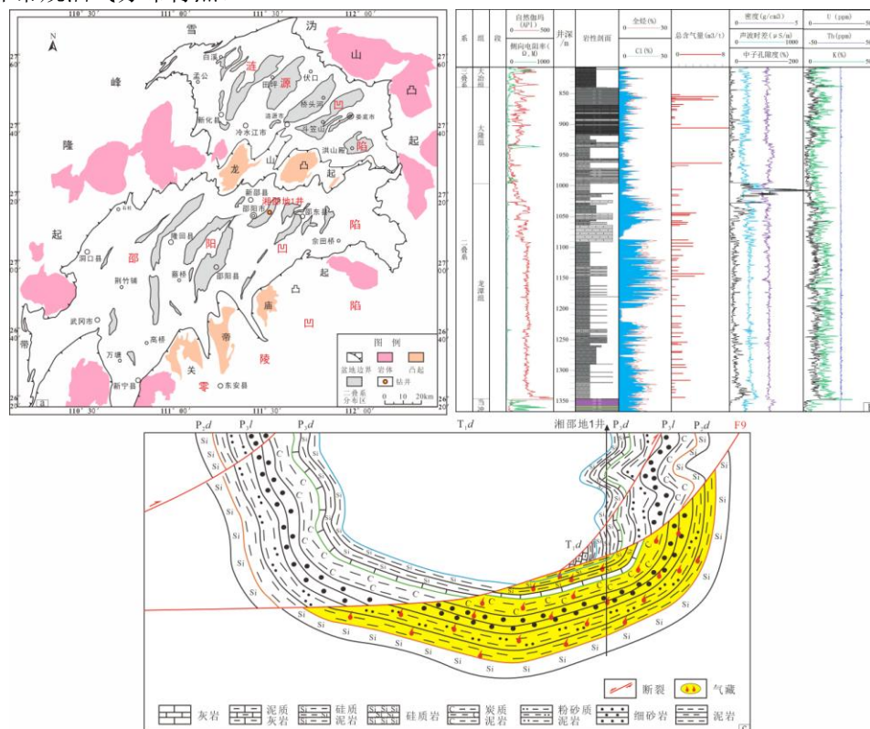
图 1 湘邵地 1 井构造位置图 (a)、主要含气层段岩性和含气性参数柱状图 (b)、以及富集模式图 (c)
