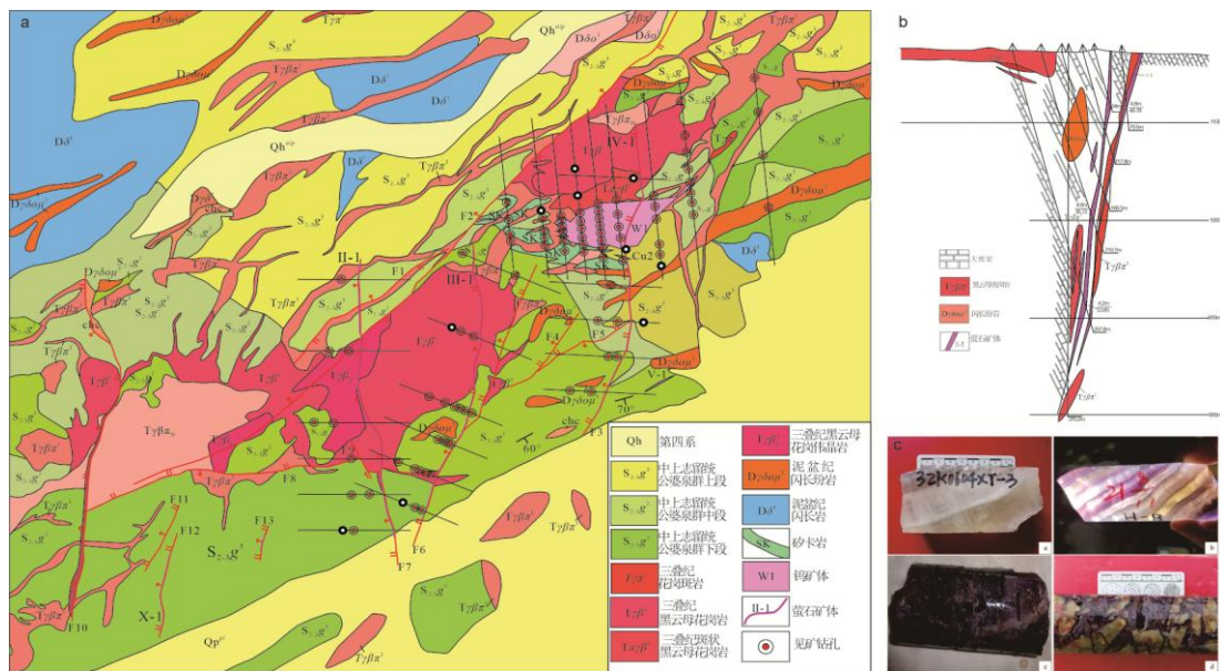
图 1 矿区地质简图 (a)、勘探线剖面图 (b) 及矿石特征 (c)
