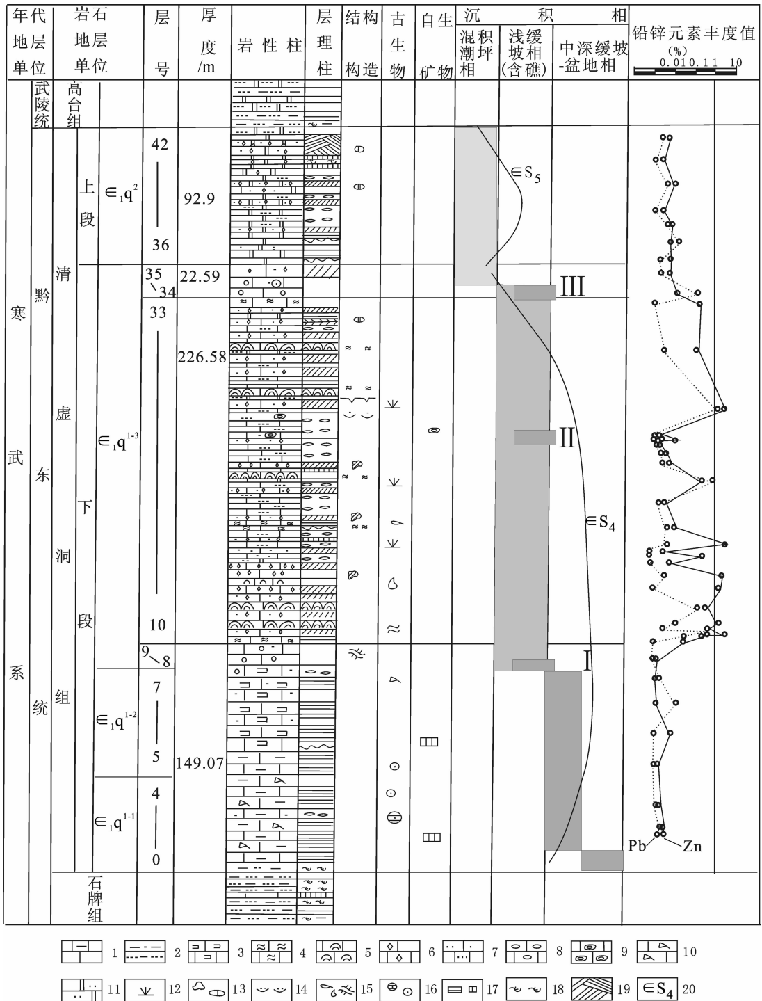
图2 贵州松桃把寨寒武系清虚洞组地层综合柱状图
