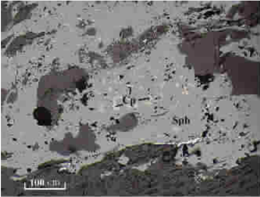
图 6 核桃坪 Pb-Zn 矿床黄铜矿和闪锌矿形成的乳浊构造
