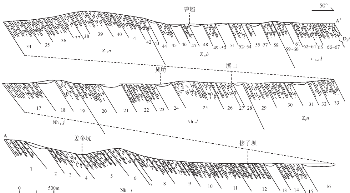
图 2 福建省长汀县楼子坝姜畚坑组(Nh 1j )、赖坑组(Nh 2l )、南岩组(Z 1n )和黄连组(Z 2h )实测剖面图
